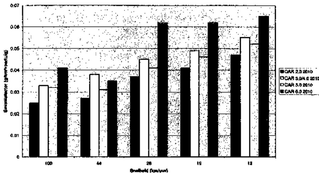
Geprognoseerde emissiefactoren PM10 per kilometer auto's 2010
