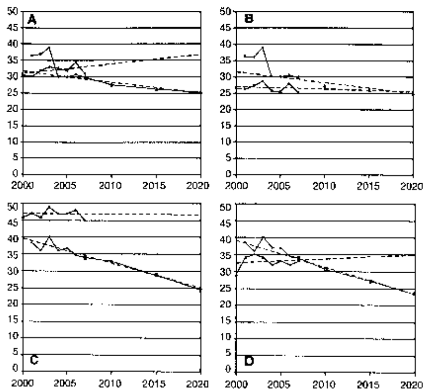
Figuur 2: Vergelijking gemeten en GCN-concentraties op de locaties van twee meetpunten (drukke straat en stadsachtergrond) in Amsterdam. (Doeke: gemeten; helder: GCN; stippollijnen: trend.)
