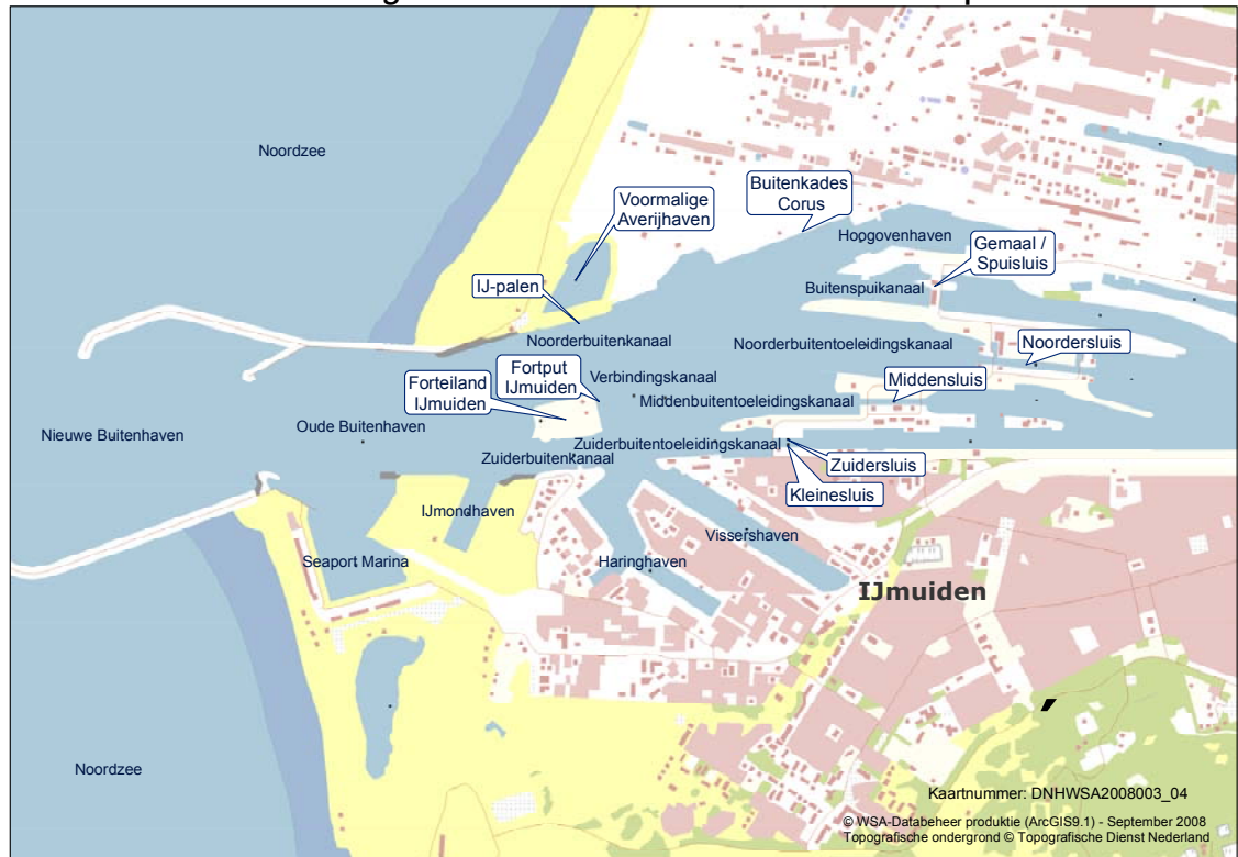
afbeelding 2.3. De havenhoofden en het sluiscomplex IJmuiden
