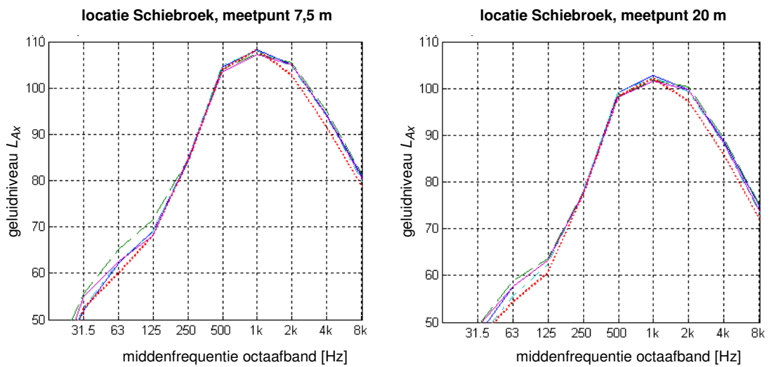
Figuur C 3.1b: A-gewogen niveaus L_{Ax} in dB(A) in octaafbanden per treinpassage richting Amsterdam, meetlocatie in Schiebroek.
