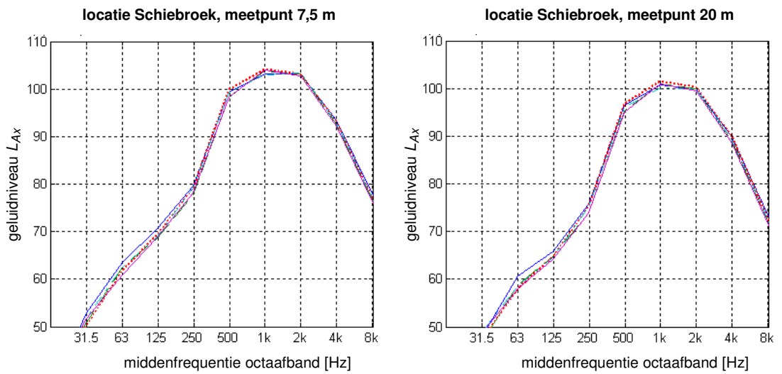
Figuur C 3.1a: A-gewogen niveaus L_{Ax} in dB(A) in octaafbanden per treinpassage richting Rotterdam, meetlocatie in Schiebroek.
