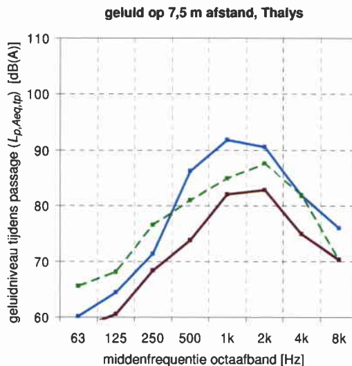
Figuur D 1.1: Gemeten geluiddrukniveau van de Thalys op 7,5 meter afstand van het spoor bij 160 km/h (blauwe lijn), vergeleken met de berekende geluiddruk voor hogesnelheidsmaterieel van categorie 9 op spoor in ballastbed conform de emissiekentallen van 2006 (groene lijn) en conform de emissiekentallen van 2009 (rode lijn).
