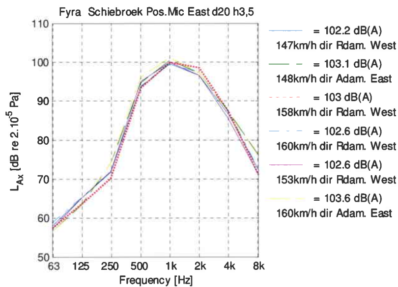
Figuur B 3.1a: A-gewogen geluidexpositieniveaus L_{Ax} in dB(A) in octaafbanden per treinpassage richting Rotterdam, westkant, meetlocatie Schiebroek , intercitymaterieel (Prioritytuigen) bij 160 km/h op 20 m uit het hart spoor aan de oostkant.
