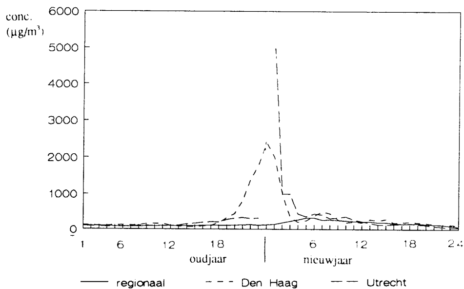
Figuur 5 De gemeten regionale concentratie fijn stof en de concentratie in steden rond de jaarwisseling. Meetreeksen die sterk beïnvloed zijn door lokale emissies (Wageningen en Braakman) zijn weggelaten bij de bepaling van de regionale concentratie.
