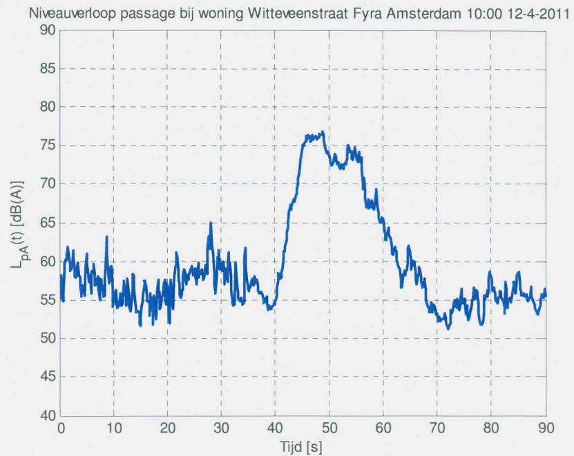
Figuur C1: Niveauperloop van de A-gewogen geluiddruk 2 meter voor de gevel van de woning aan de Witteveenstraat, voor een Traxx/Prio passage, richting Amsterdam, op 12 april 2011 om 10:00.
