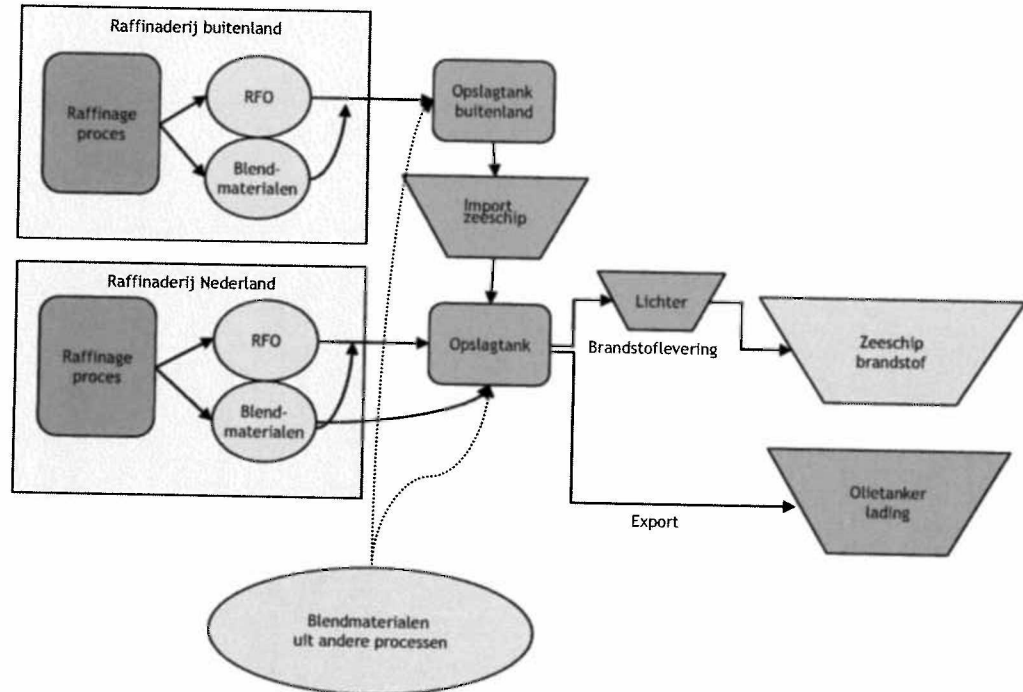
Figuur 8 Eenvoudige schets bunkerolieketen
