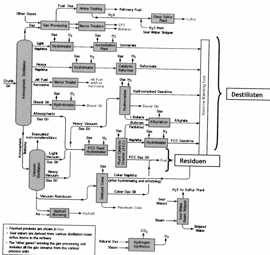
Figuur 10 Typerende schets van een moderne raffinaderij
