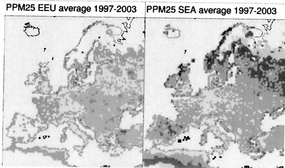
Figuur 11 Bijdragen zeescheepvaart aan fijn stof (PM 2,5 ) concentraties in Europa
