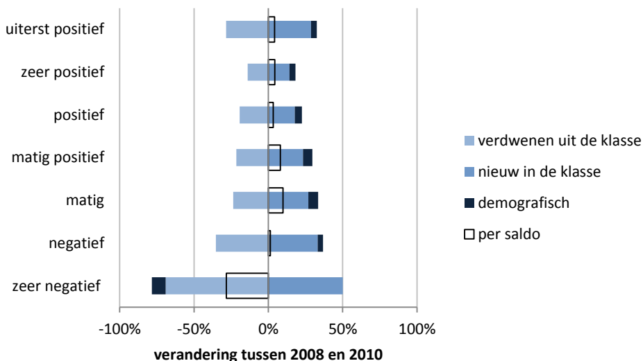
figuur 5-2 Ontwikkeling van het aantal inwoners per klasse tussen 2008 en 2010
