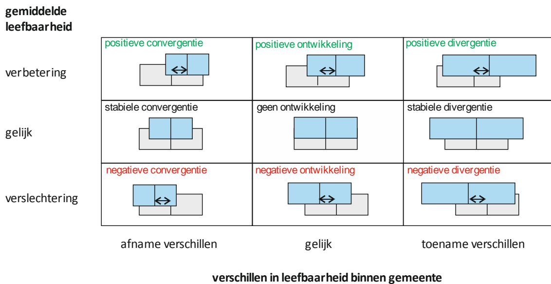
figuur 5-8 Soorten ontwikkelingen, naar verandering van het gemiddelde en verandering van de spreiding
