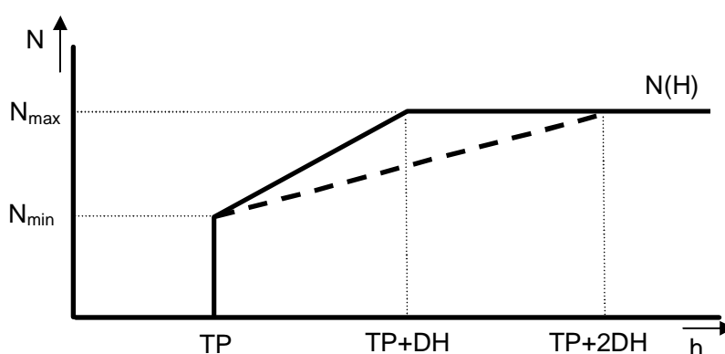
Figuur C.0.1 Het aantal slachtoffers, gegeven een overstroming, als functie van de waterstand.
