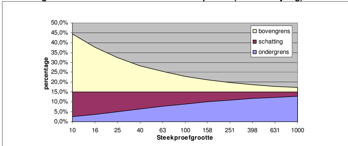
Afbeelding 3.22. Betrouwbaarheidsinterval voor q = 0.15 (>20 % afwijking)
