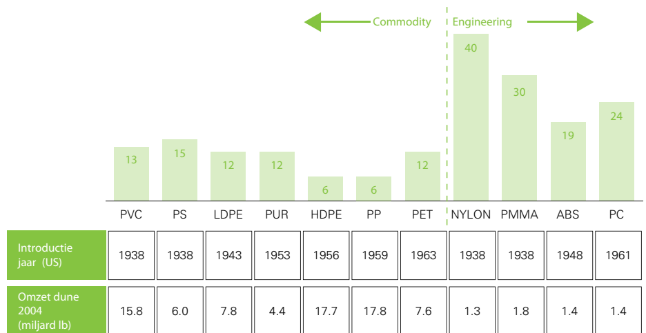
Figuur 51: Gemiddelde duur om een jaarlijkse verkoop van 136.000 ton polymeer te realiseren per productiefaciliteit
