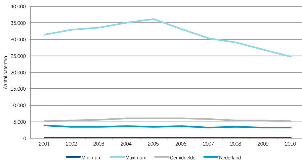
Figuur 34: EPO-octrooiaanvragen, 2001-2010
