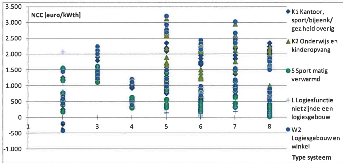
Figuur 7 Netto contante meerkosten van koel- of verwarmingssystemen in bestaande utiliteitsgebouwen, calculatieperiode=20 jaar
