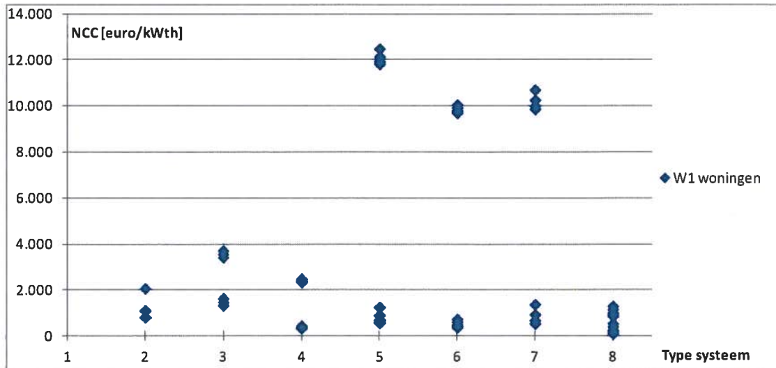
Figuur 6 Netto contante meerkosten van koel- of verwarmingssystemen in bestaande woningen
