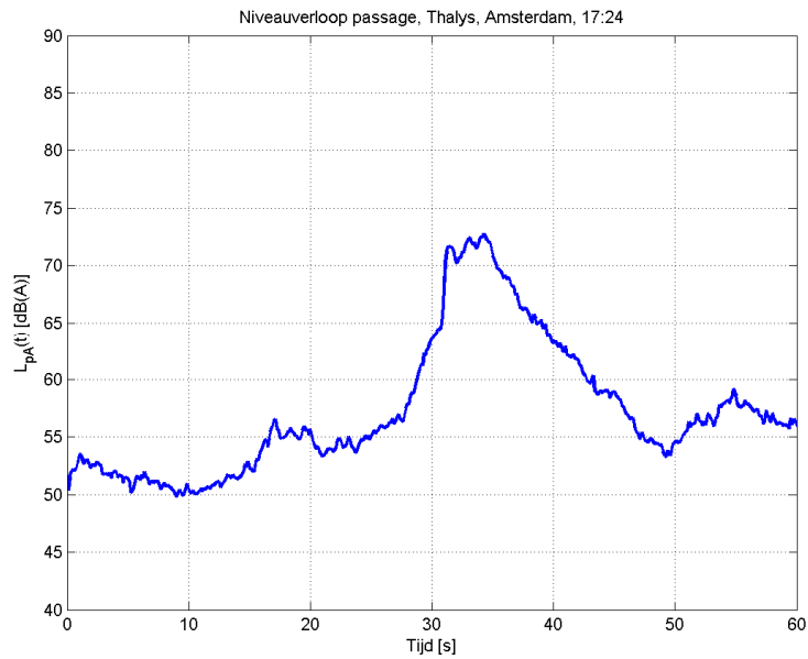
Figuur B9 Niveauperloop van de A-gewogen geluiddruk naast de woning aan de Berkelseweg voor een Thalys passage, richting Amsterdam, op 14 november 2012 om 17:24.
