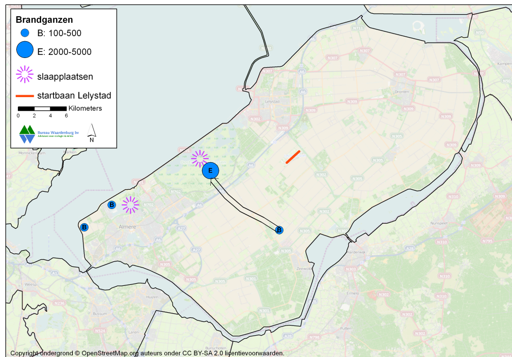
Figuur 3.5 Overzicht pleisterplaatsen van ganzen ( Branta soorten) en de bijbehorende vliegbanen van en naar slaapplaatsen. Bronnen: Koffijberg et al. 1997, Van Roomen et al. (2007), Voslammer et al. (2004) en www.sovon.nl .
