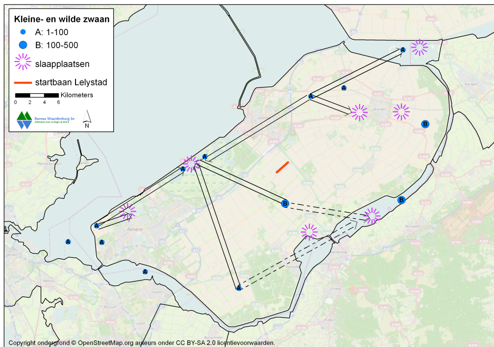
Figuur 3.3 Verspreiding van kleine en wilde zwanen. Weergegeven zijn de pleisterplaatsen, slaapplaatsen en (mogelijke) vliegbanen. Bronnen: Koffijberg et al. (1997) en Van Roomen et al. (2007) en www.sovon.nl .
