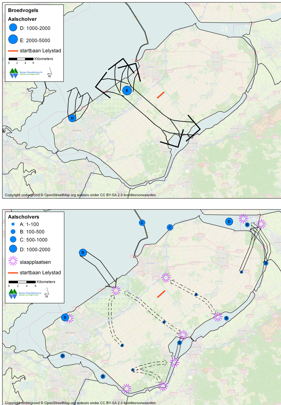
Figuur 3.1 Verspreiding aalscholvers: broedvogels (boven) en niet-broedvogels (onder). Boven zijn de aantallen broedvogels en bijbehorende vliegbanen weergegeven. Onder zijn de aantallen pleisteraars, (mogelijke) slaapplaatsen en de bijbehorende (mogelijke) vliegbanen weergegeven. Bronnen: Van Roomen et al. 2007, eigen waarneming, pers. med. S. van Rijn en www.sovon.nl ,
