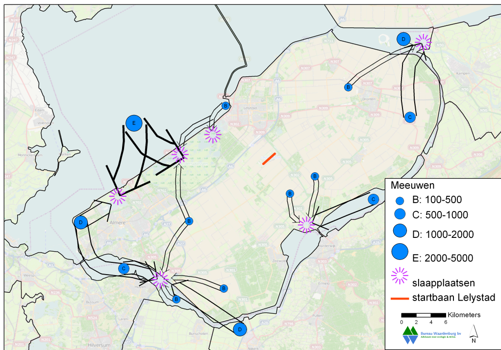
Figuur 3.9 Overzicht pleisterende meeuwen in het winterhalfjaar. Verder zijn weergegeven de (mogelijke) slaapplekken en bijbehorende (mogelijke) vliegbanen. Bronnen: Jonker & Majoor (1995), Van Roomen et al. (2007) en www.sovon.nl .
