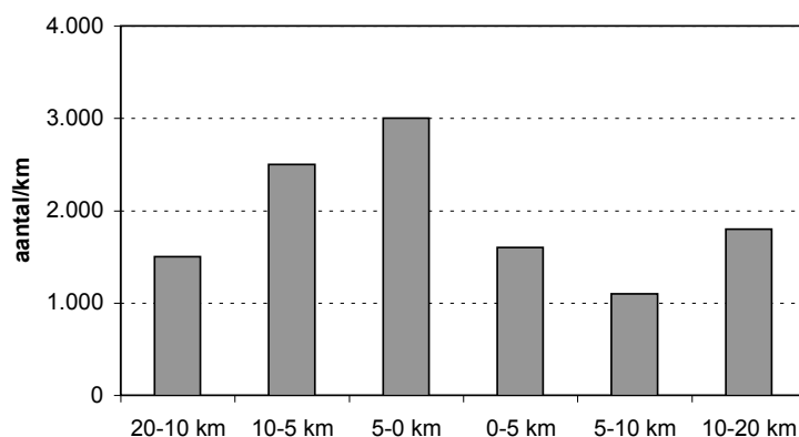
Figuur 4.1 Aantal dagelijkse bewegingen op verschillende afstanden van het vliegveld. Aantallen hebben betrekking op de orde grootte van maxima gedurende het jaar.
