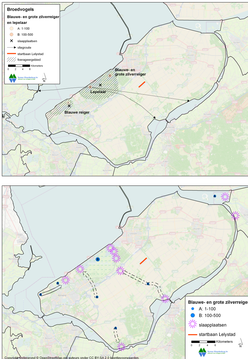
Figuur 3.2 Verspreiding van de blauwe reiger en de grote zilverreiger. Broedseizoen (boven): aantallen broedvogels en bijbehorende vliegbanen. Buiten broedseizoen (onder): de aantallen pleisteraars, (mogelijke) slaapplaatsen en de bijbehorende (mogelijke) vliegbanen van reigers. Lepelaars delen in deze vliegbewegingen. Bronnen: Boele et al. (2011), Van Roomen et al. (2007) en www.sovon.nl .
