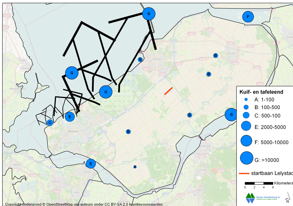
Figuur 3.7 Dagrustplaatsen van de kuif- en tafeleend. Daarnaast zijn de vliegbewegingen weergegeven van enkele dagrustplaatsen in natuurgebieden (zie verder hoofdstuk). Bronnen: Van Roomen et al. (2007) en www.sovon.nl .
