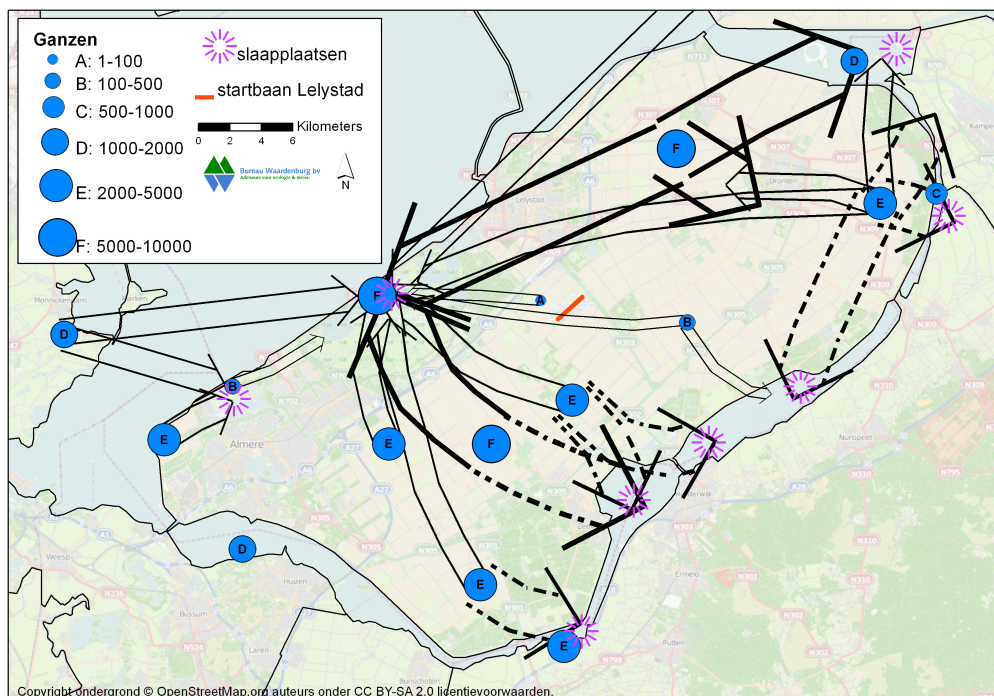
Figuur 3.4 Overzicht pleisterplaatsen van ganzen (Anser soorten) en de bijbehorende (mogelijke) vliegbanen van en naar slaapplaatsen. De slaapplaatsen weergegeven op de randmeren zijn mogelijk in gebruik. Bronnen: Koffijberg et al. 1997, Van Roomen et al. (2007), Voslamber et al. (2004) en www.sovon.nl .
