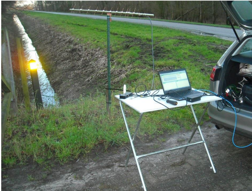
Figuur F.1: Meetopstelling richtantenne op één van de meetlocaties
