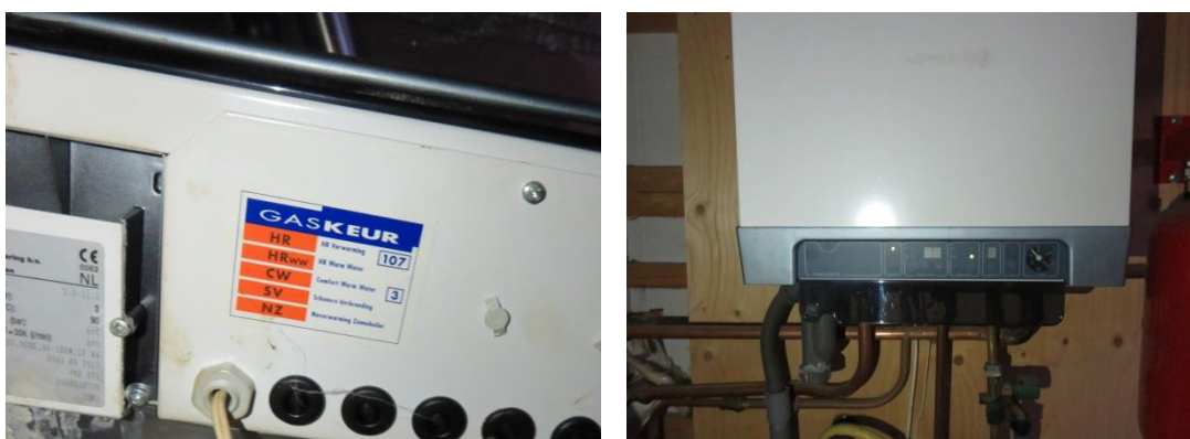
Figuur 16: CV-ketel woning 42
