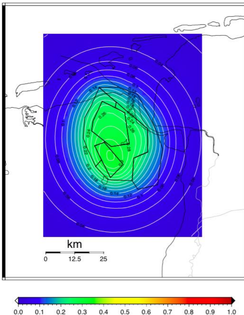
Figuur 4: Peak Ground Acceleration (PGA) contouren voor een herhalingsjijd van 475 jaar met 21 bevingen per jaar.
