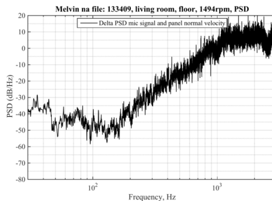
Figuur VI.6 Voorbeeld grafiek afstralefficiëntie (Melvin na maatregelen)
