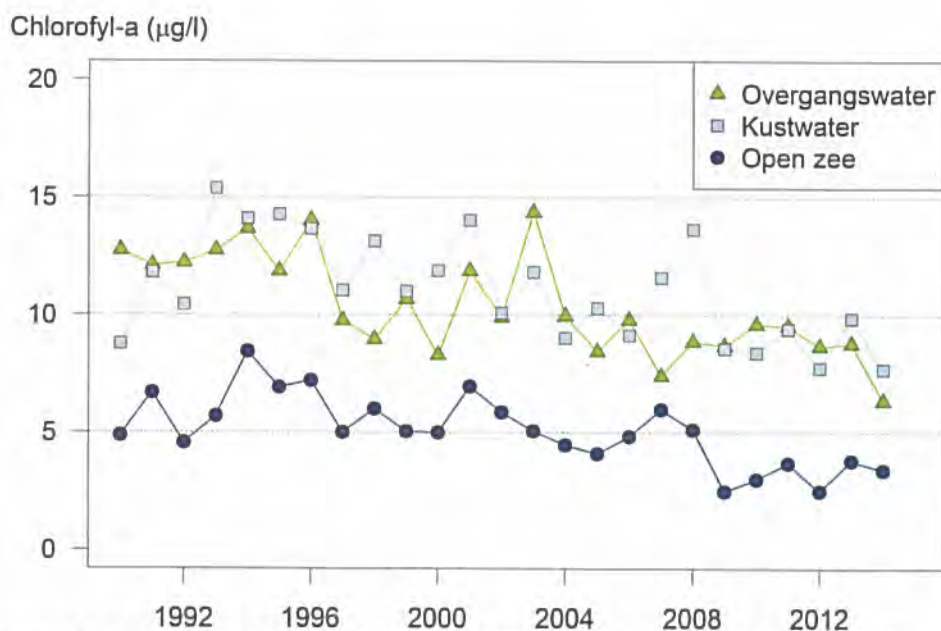
Figuur 7.4 Gemiddelde chlorofyl-a-concentratie (µg/l) in de zomer op open zee en in de Nederlandse overgangs- en kustwateren in de periode 1990-2014
