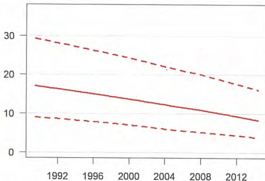
Figuur 6.8 Berekende trend in de nitraatconcentratie (wintergemiddelde als NO 3 in mg/l) voor de regionale KRW-wateren; mediaan (doorgetrokken lijn) en 25- en 75-percentiel (gestippelde lijnen)
