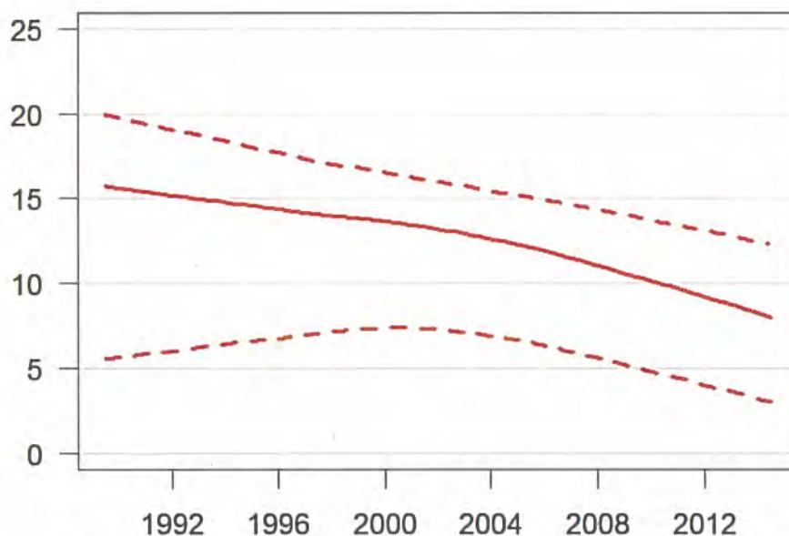
Figuur 7.5 Berekende trend voor de nitraatconcentratie (wintergemiddelde als \text{NO}_3 in mg/l) voor de KRW-overgangswateren; mediaan (doorgetrokken lijn) en 25- en 75-percentiel (gestippelde lijnen)
