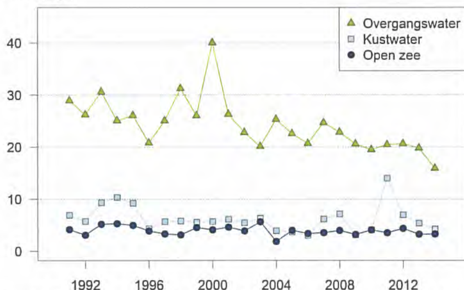
Figuur 7.2 Maximum nitraatconcentratie (als \text{NO}_3 in mg/l) op open zee en in de Nederlandse overgangs- en kustwateren in de winter in de periode 1991-2014
