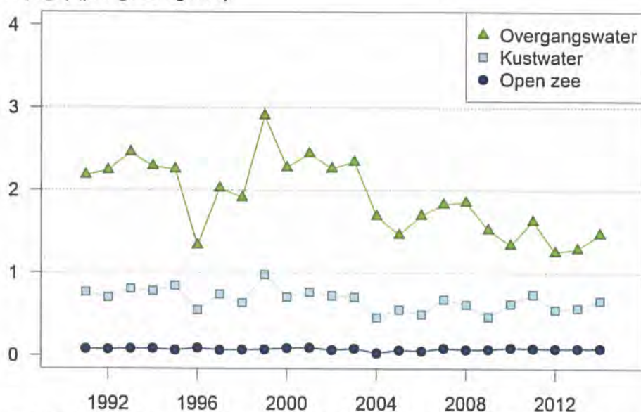
Figuur 7.3 Gemiddelde opgeloste anorganische stikstofconcentraties in de winter (DIN, als N in mg/l), gestandaardiseerd voor een saliniteit van 30 psu, in de Nederlandse overgangswateren, kustwateren en open zee in de periode 1991-2014
