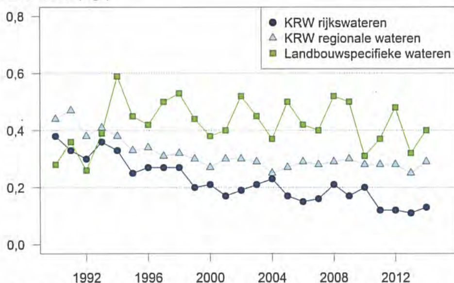
Figuur 6.6 Totaal-fosforconcentratie (zomergemiddelde als P in mg/l) in zoete wateren in de periode 1990-2014
