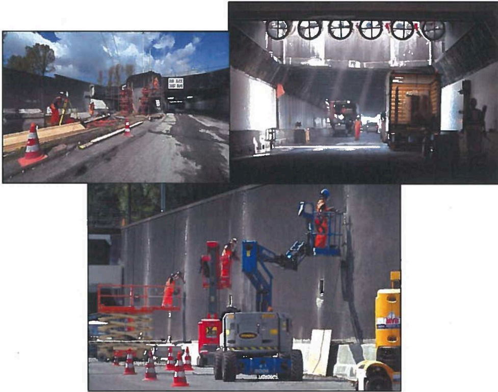
Figuur 8.3 Beelden van de renovatie van de Velsertunnel
