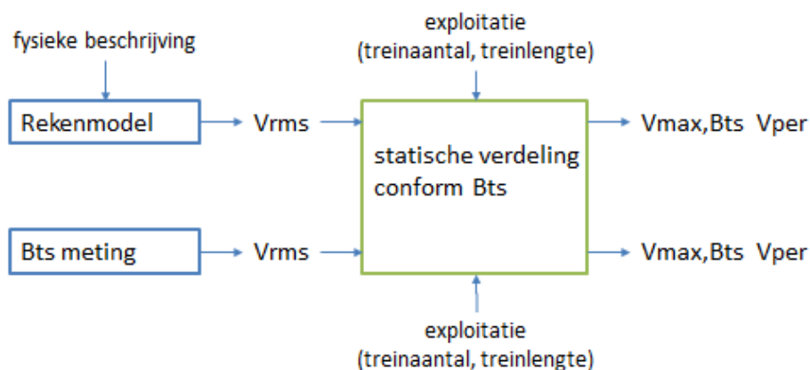
Figuur 9 Schematische weergave rekenmodel, rekengrootheden en normgeving.
