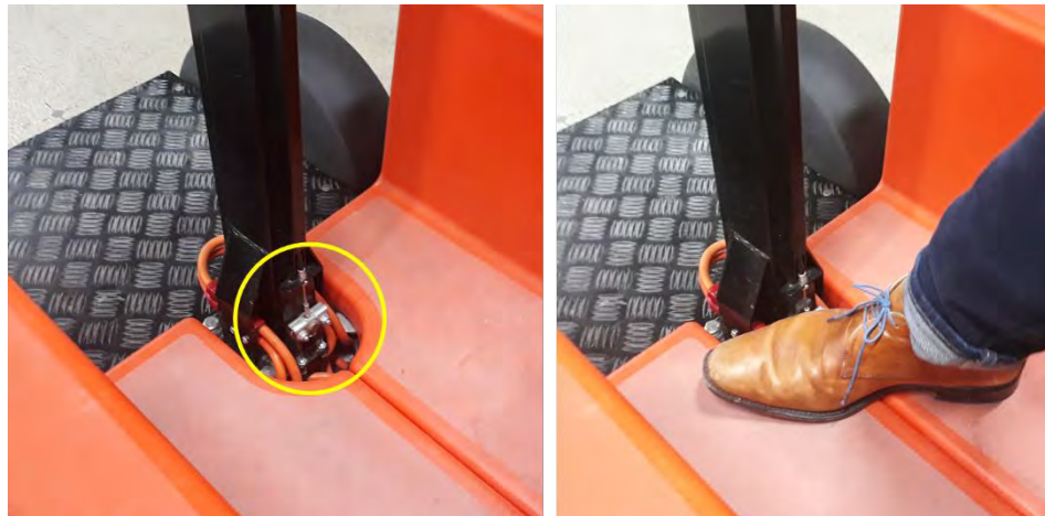
Figuur 11: Nieuw model Stint onbeschermd rembediening.
