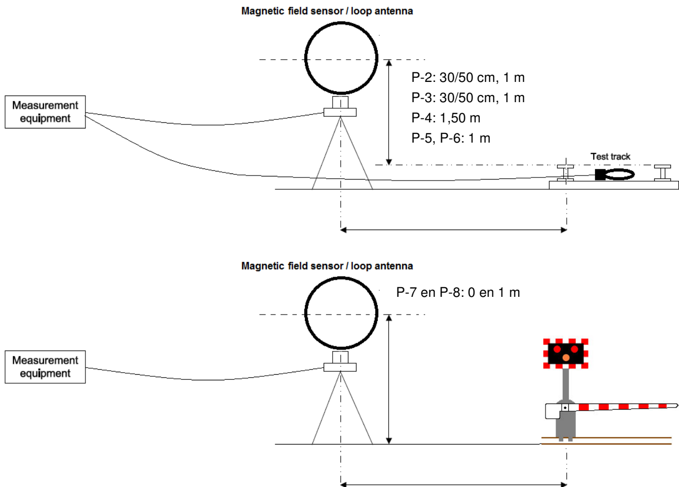
Figuur 4.2-1: Testopstellingen
