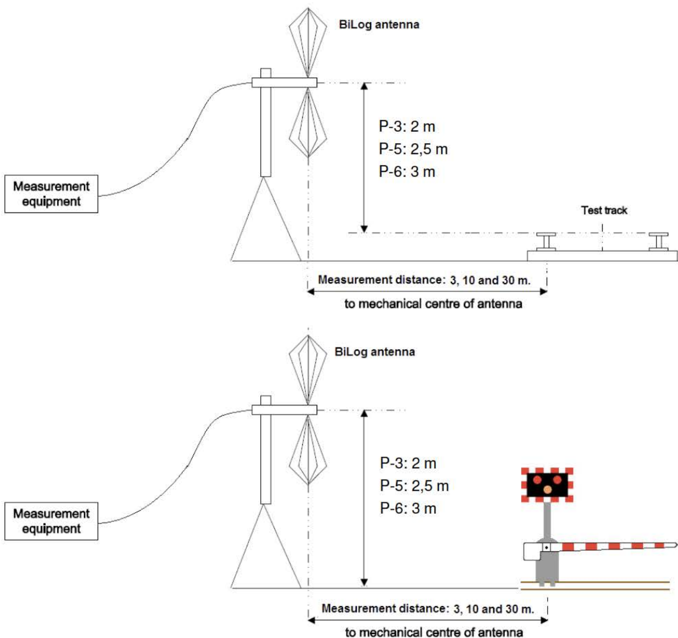
Figuur 4.3-1: Testopstellingen.
