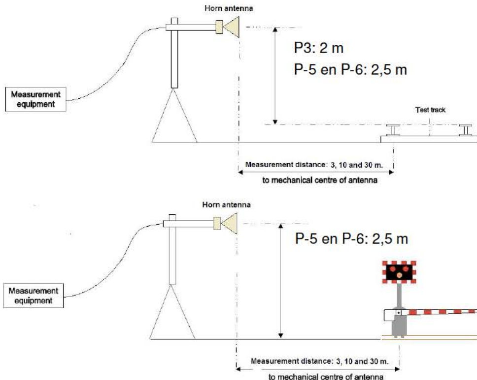
Figuur 4.4-1: Testopstellingen.
