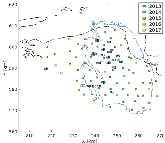
Figuur 1: Het versnellingsmeternetwerk in Groningen
