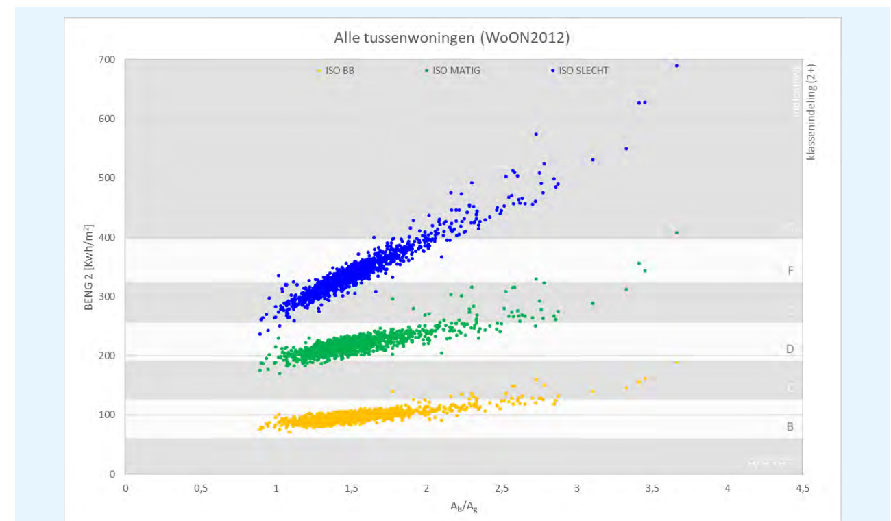
figuur 3: relatie A_{15}/A_g en BENG 2 bij alle tussenwoningen WoON 2012 met indicatieve labelklasse-indeling 2+
