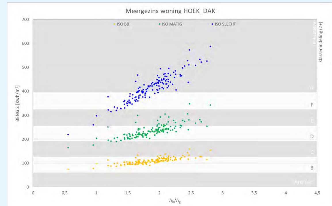
figuur 17: Spreiding A10/Ag en BENG 2 meergezinswoning HOEK_DAK
