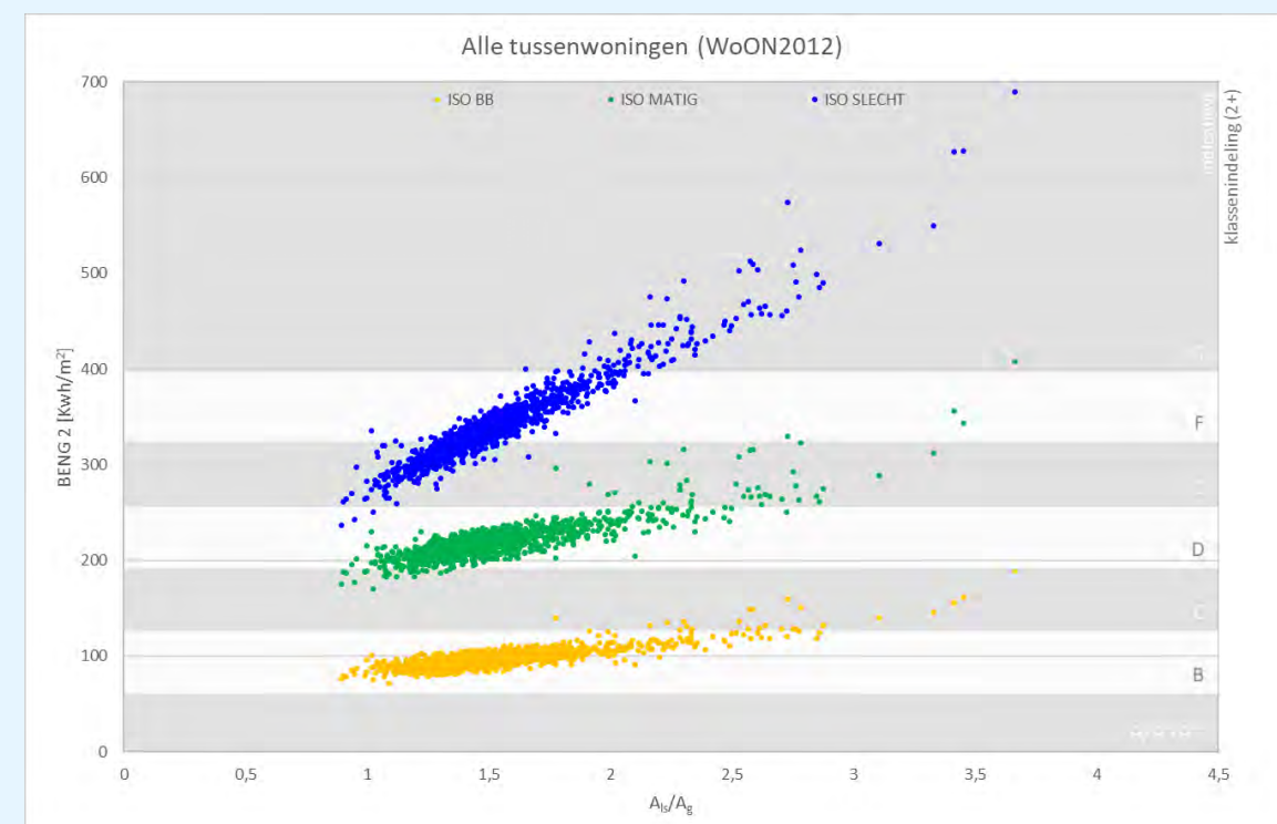
figuur 18: Spreiding A10/Ag en BENG 2 tussenwoning
