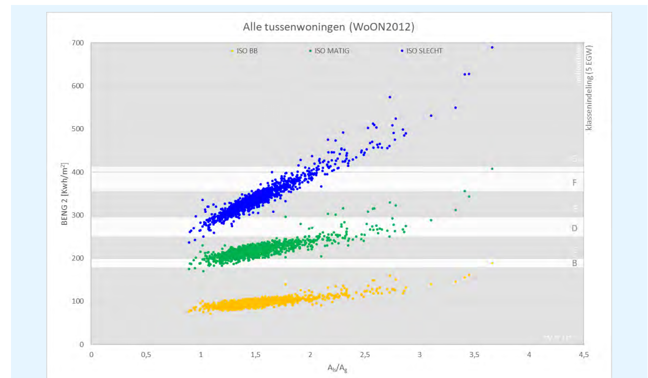
figuur 4: relatie A_{15}/A_g en BENG 2 bij alle tussenwoningen WoON 2012 met indicatieve labelklasse-indeling 5 (egw)
