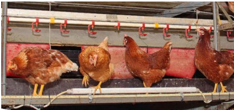
Figuur 3.2 Mite Alert, automatische vogelmijt monitoringssysteem in de stal.
