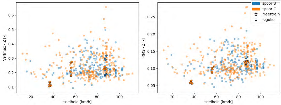
Afbeelding V.17 Spreidingsdiagram van snelheid met trillingsniveau voor passages bij meetopstelling S3-3 met kleurstelling naar spoor, en indicatie voor meetrein
