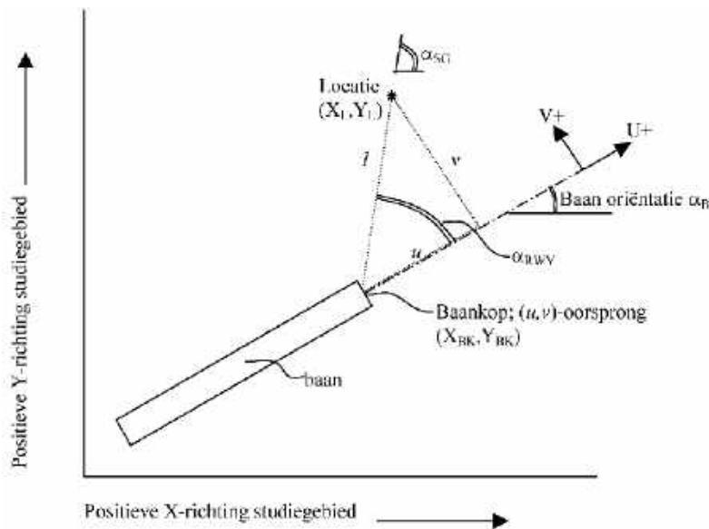
Figuur 3 Baantransformatie
