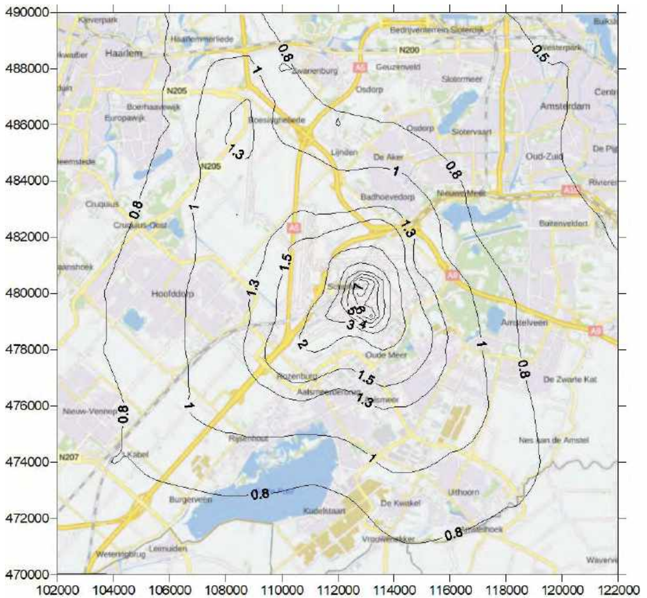
Figuur K.52: Contourplot (20 x 20 km) van de 99,9 percentiel VOS scenario 500k_NNHS (2020) in ouE/m^3
