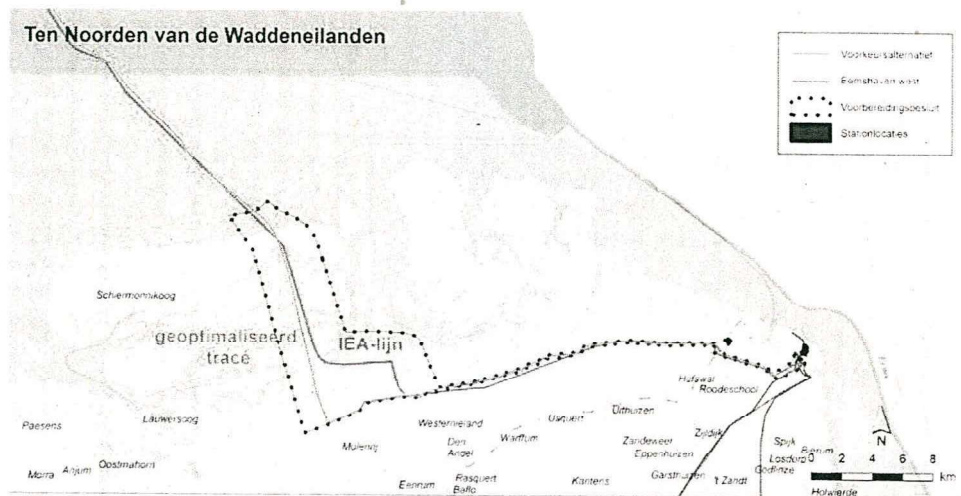
Overzicht voorkeursalternatief Eemshaven west met zoekstrook en inclusief de twee opties voor een transformatorstation
