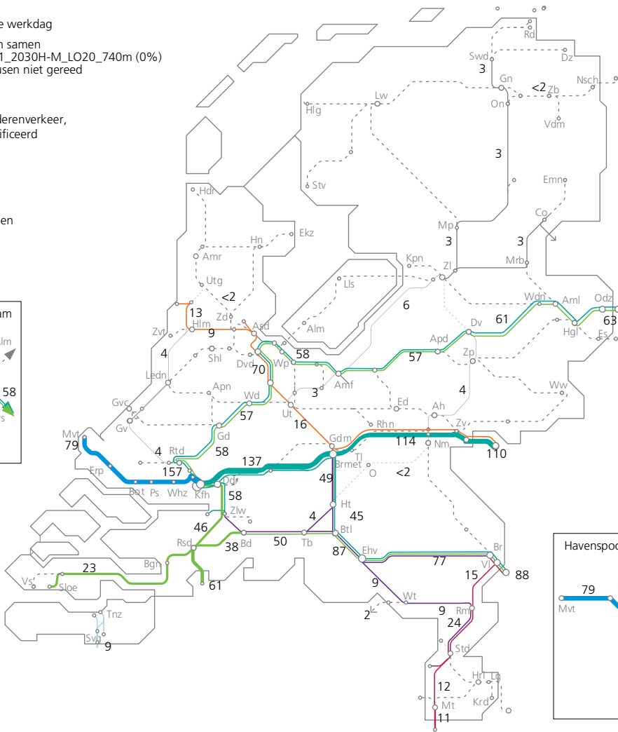
Figuur G.2.10: Aantal goederentreinen en -paden in 2030 Hoog als 3e spoor Zevenaar – Oberhausen niet gereed is
