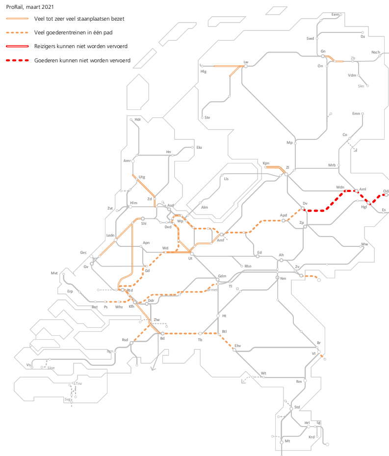
Figuur 7.2.1: Capaciteitsanalyse Reizigers en Goederen 2040 Hoog
