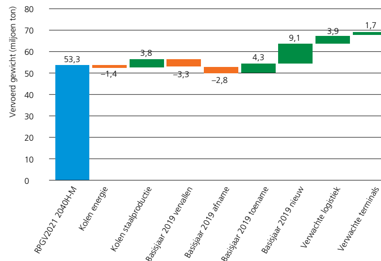
Figuur F.2: Wateranalyse verrijking prognose spoorgoederenvervoer voor het hoge scenario 2040
