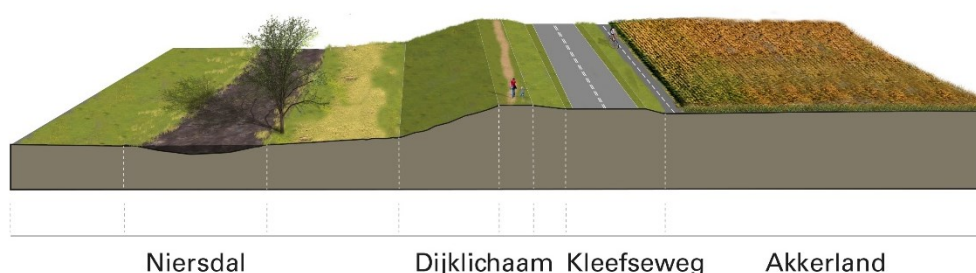
Afbeelding 28: Perspectiefdoorsnede dijkversterking Kleefseweg nabij Maria Roepaen in deelgebied Niersdal
