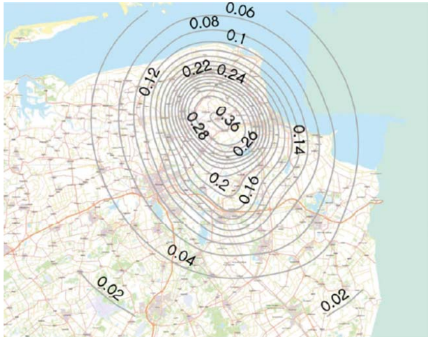
Figuur 6.1 Kaart met grondversnellingen van het KNMI
