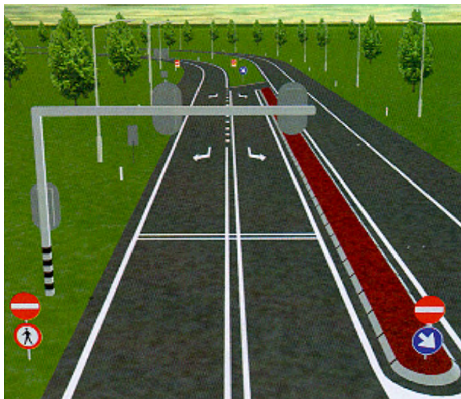
Afbeelding 4.3. Correctieweg die ervoor zorgt dat een automobilist die de afrit in plaats van de toerit oprijdt, automatisch naar de toerit wordt geleid. De rijstrook voor verkeer dat afslaat naar links, gaat in de andere richting via een doorsteek over in de toerit (Bron: RWS Zuid-Holland/Grontmij in Brevoord, 1998).
