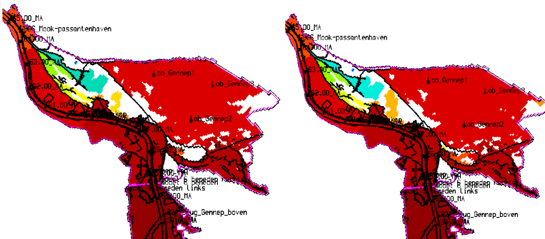
Figuur 41. Absolute waterstand voor de referentie (norm, V1) en afwijkingen ten opzichte van de legger (V2a, ongesaldeerd). In beide gevallen stroomt de Lob van Genneep in ongeveer gelijke mate in.
