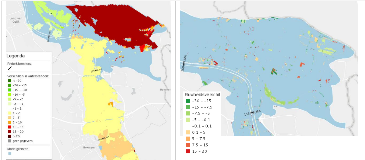
Figuur 40. Waterstandsverschil Maas bij Lob van Genneep (links) en ruwheidsverschil (rechts).
