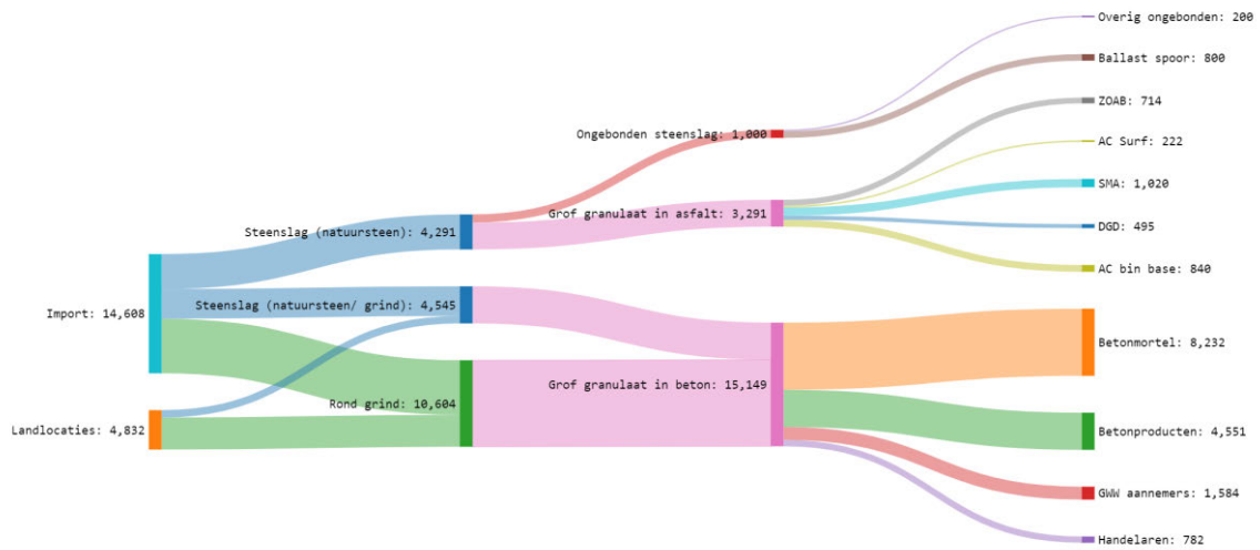
Afbeelding 5 Sankey diagram van het gebruik van grind en steenslag in het basisjaar 2019, uitgedrukt in kilotonnen.
