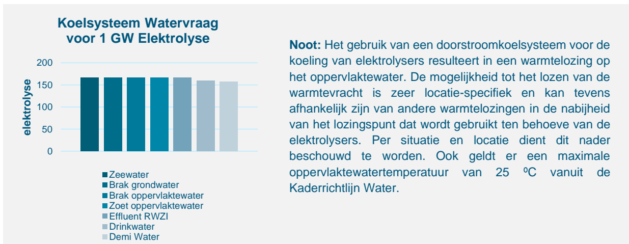
Figuur 3-8: Grafische weergave van de watervraag per waterbron voor gebruik in doorstroomkoelsystemen
