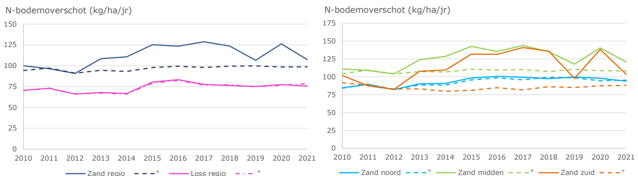
Figuur 3.7a Berekend verloop van het N-bodemoverschot (kg/ha/jr.) van landbouwgronden in de zand- en lössregio (links) en in 3 zandgebieden (rechts). Getrokken lijnen geven de situatie weer bij plaatsing van 'te plaatsen dierlijke mest' en stippellijnen geven de situatie weer bij bemesting binnen de gebruiksruijme.
