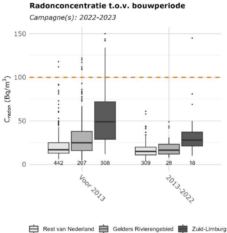
Figuur 4.8 Boxplots van de gemeten radonconcentraties voor woningen die gebouwd zijn voor en na 2013, voor Zuid-Limburg, het Gelders Rivierengebied en de rest van Nederland. Onder iedere boxplot staat het aantal meetpunten. De radonconcentratie is het laagst in woningen die gebouwd zijn sinds de vorige survey in 2013-2014. De oranje stippellijn geeft het Nederlands referentieniveau weer. De y-as is afgekapt op 150 Bq/m 3 , 21 meetpunten zijn niet weergegeven.
