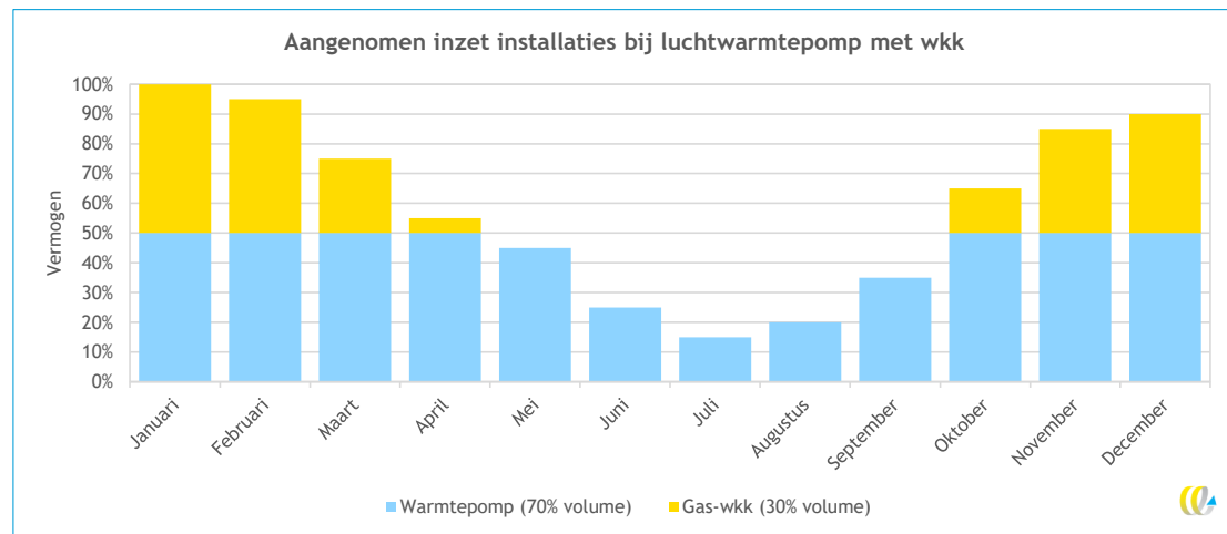
Figuur 26 - Voorbeeld aangenomen dimensionering installaties
