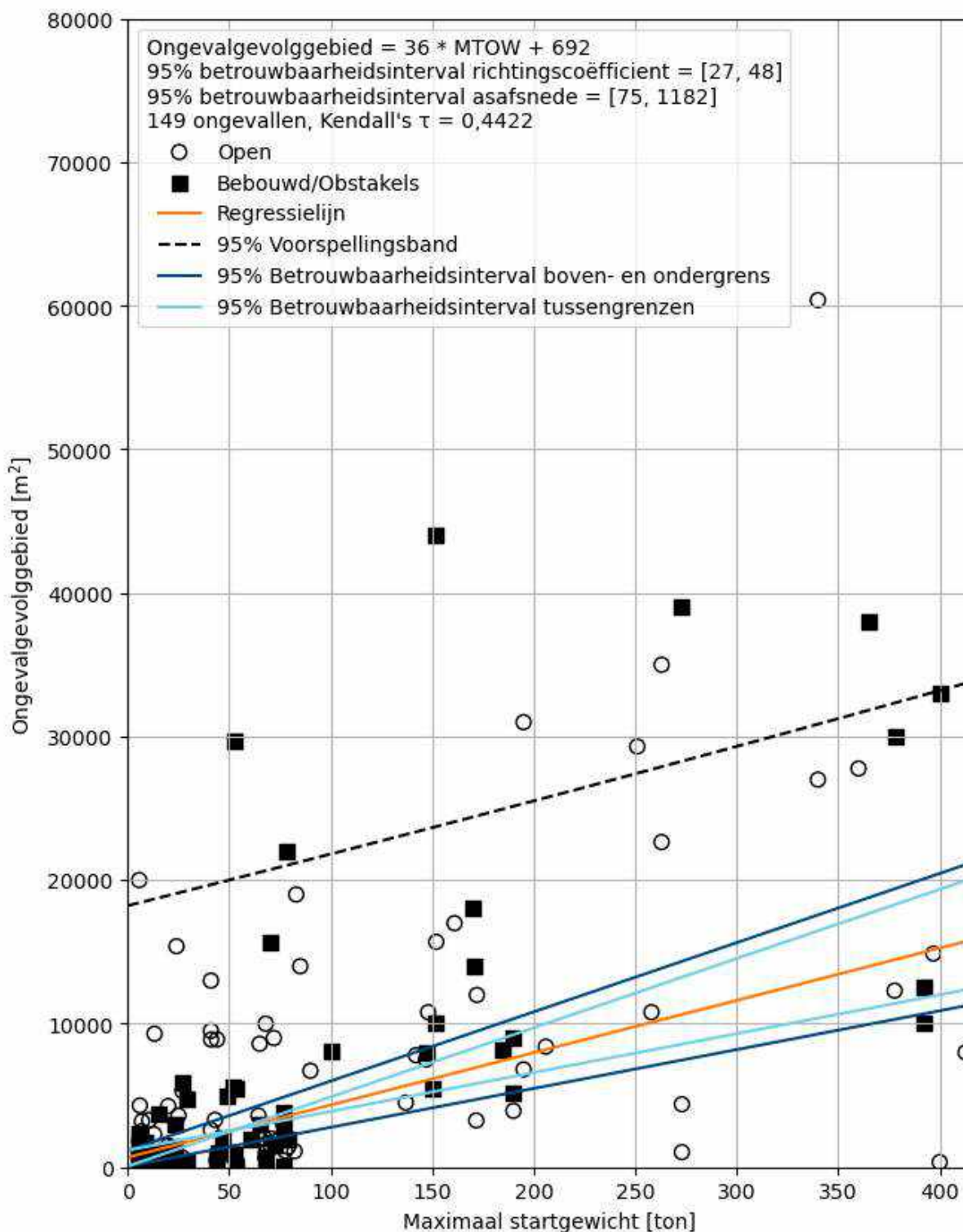
Figuur 5-5: Grafiek met Kendall Theil Sen regressie en y = a \cdot x + b (MTOW = maximaal startgewicht). De tussengrenzen tonen een combinatie van de hoogste constante en laagste richtingscoëfficiënt en omgekeerd
