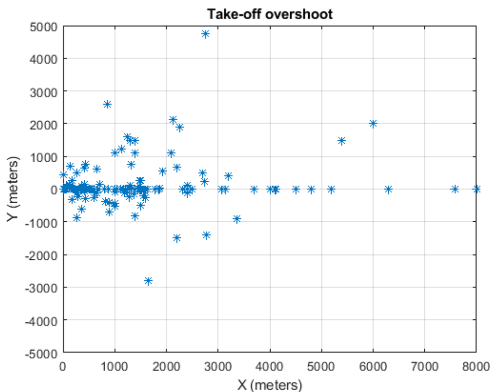
Figuur 3-1: Scatterplot van Take-off overshoot. Opmerking: één datapunt is geclassificeerd als outlier met |y| > 4000\text{m}
