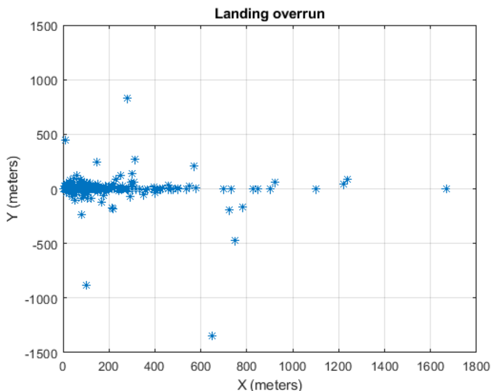
Figuur 3-4: Scatterplot van Landing overrun. Opmerking: drie datapunten zijn geclassificeerd als outliers ( |y| > 500\text{m} )
