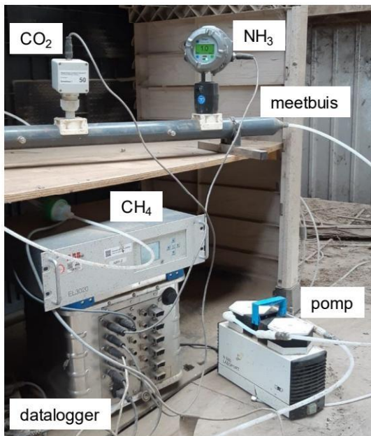
Figuur 3.2 Meetopstelling WLR voor continue metingen.
