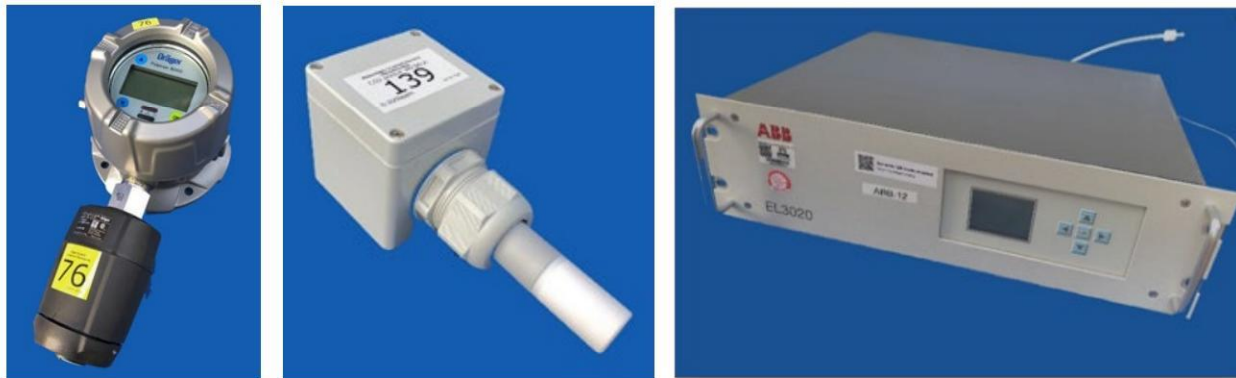
Figuur A1 Links: Dräger Polytron 8000 met de FL-6813260 sensor voor \text{NH}_3 -concentratiemetingen. Midden: Vaisala CARBOCAP® met GMP252 sensor voor \text{CO}_2 -concentratiemetingen. Rechts: ABB EasyLine EL3000 met Uras26 sensor voor \text{CH}_4 -concentratiemetingen.
