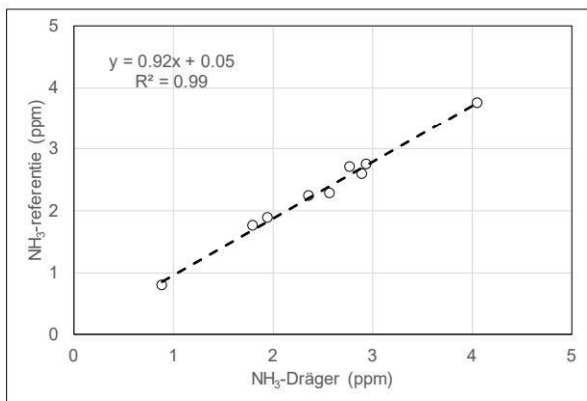
Figuur 3.4 Voorbeeld van regressielijn (veldkalibratie) van een van de \text{NH}_3 Dräger-sensoren in de praktijk.
