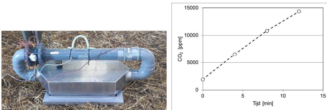
Figuur A5 Boxmetingen (bij geitenstallen) om de \text{CO}_2 -productie uit de pot te bepalen. Links: meetopstelling. Rechts: voorbeeld van toename in \text{CO}_2 -concentratie
