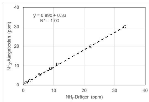
Figuur 3.3 Links: Meetopstelling voor de kalibratie van NH 3 Dräger-sensoren in het Air Quality Laboratorium (AQL) van Wageningen Livestock Research (WLR). Rechts: voorbeeld regressielijn (labkalibratie) voor één van de NH 3 Dräger-sensoren.
