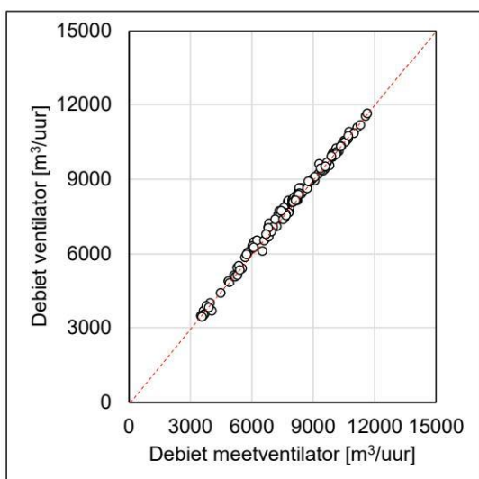
Figuur A9 Vergelijking tussen een directe bepaling van het ventilatiedebiet met meetwaaiers, en registratie via de klimaatcomputer, bij een blankvleeskalverstal (VKB1).
