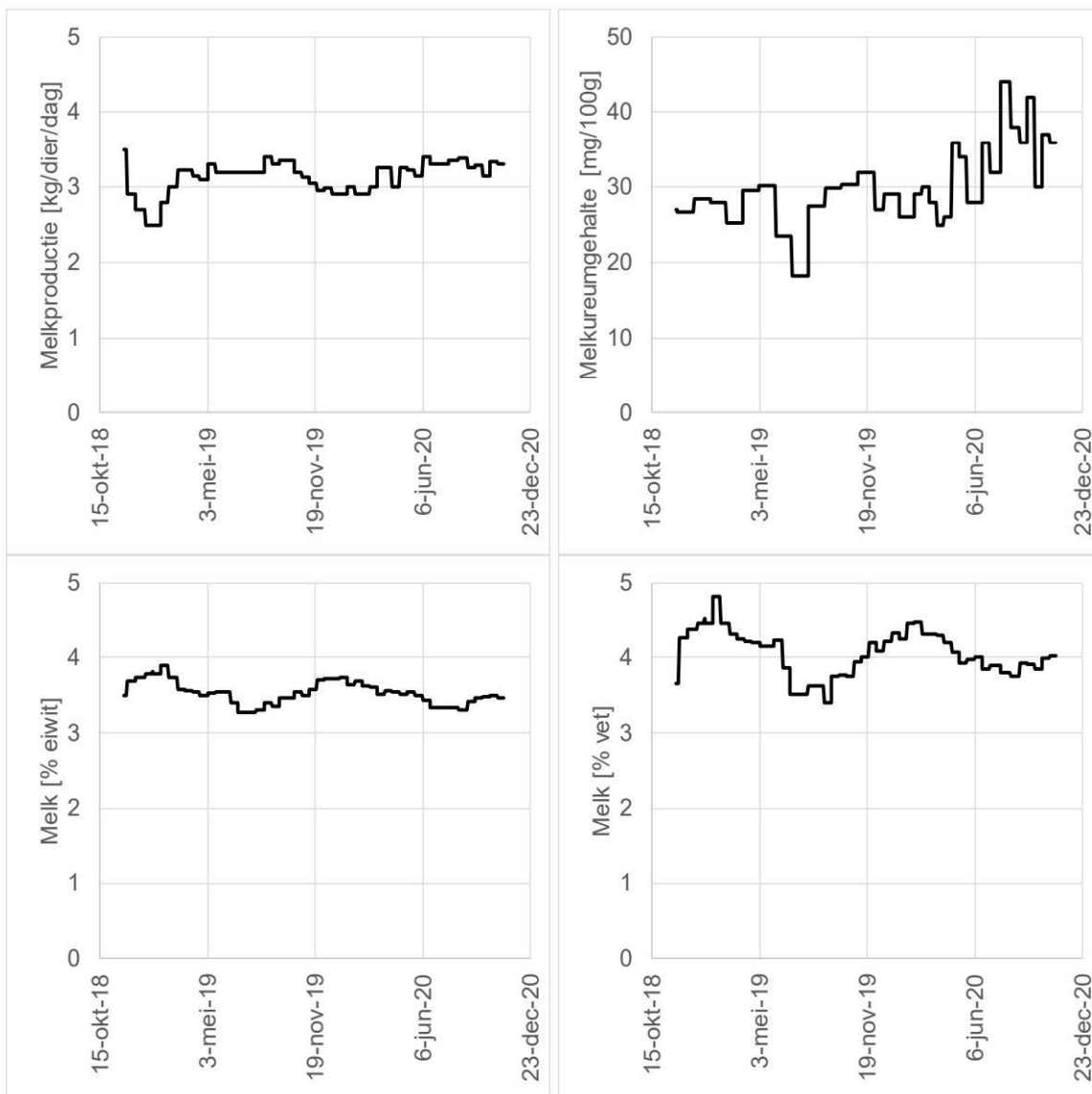
Figuur G1.2 Melkproductie en -samenstelling (2-weken basis) over de gehele meetperiode
