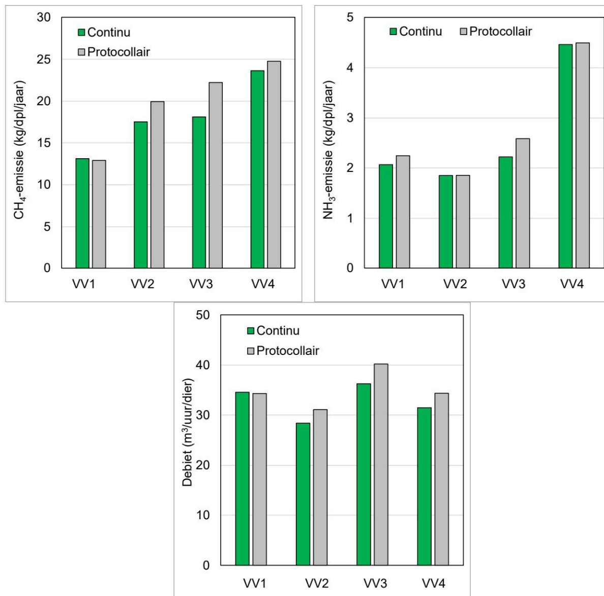
Figuur 7.2.3 Per vleesvarkensbedrijf, gemiddelde ventilatiedebiet en gemiddelde emissies van NH 3 en CH 4 voor de continue en de protocollaire metingen, wanneer gebruikt wordt gemaakt van alle beschikbare waarnemingen.
