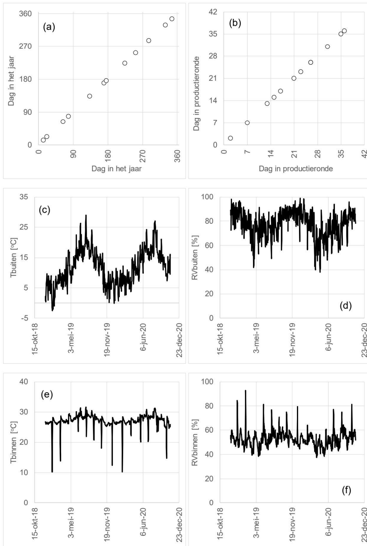
Figuur BG1.1 a) Verdeling van de metingen over de seizoenen; b) Verdeling van de metingen over een productieronde; c) t/m f) Continue metingen van een aantal klimaatparameters. T: temperatuur; RV: relatieve vochtigheid.
