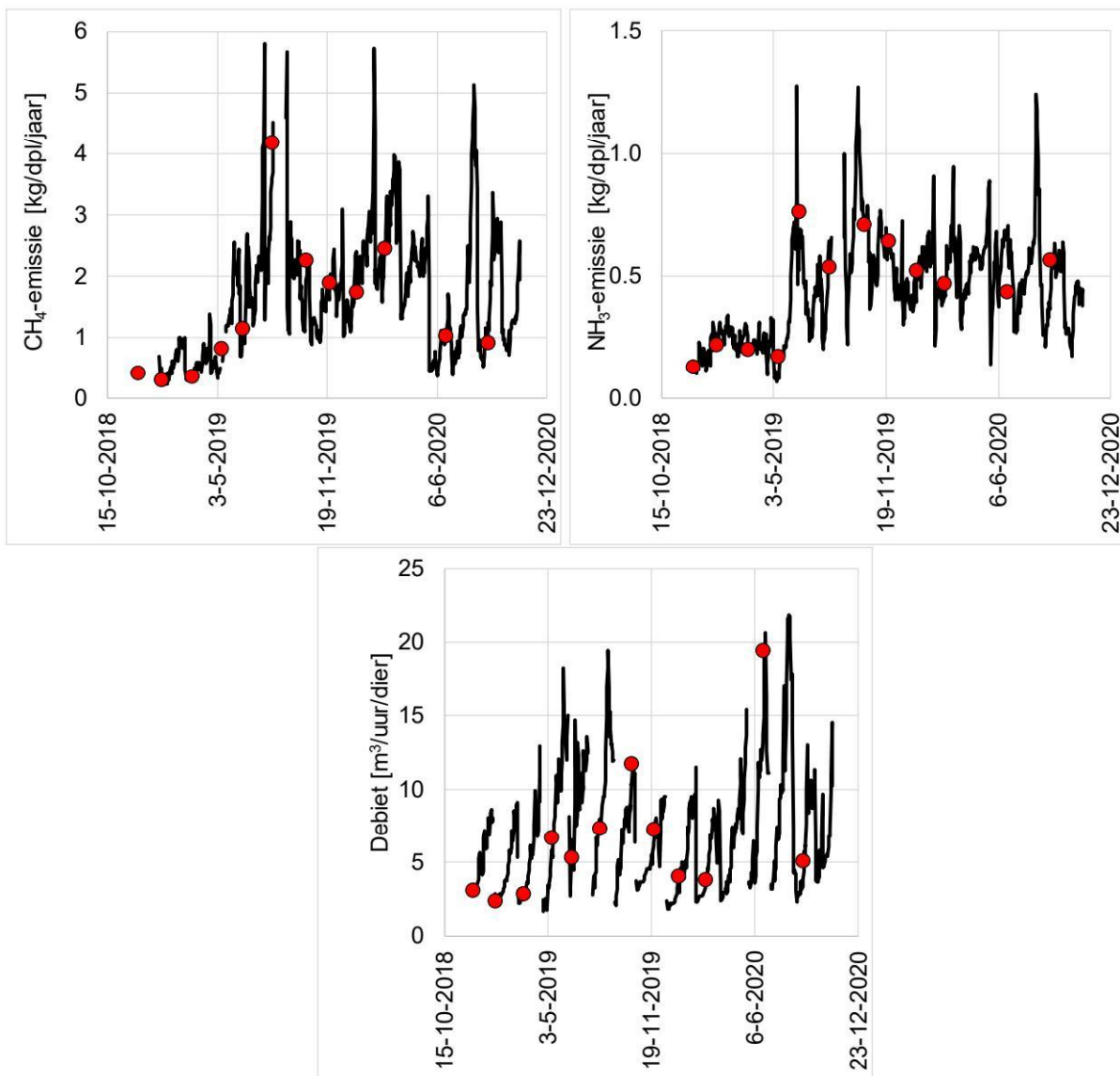
Figuur BG1.2. Linksboven: CH 4 -emissie [kg/jaar per dierplaats]; Rechtsboven: NH 3 -emissie [kg/jaar per dierplaats]; Onder: Ventilatie-debiet [m 3 /uur/dier]. De protocollaire metingen worden met rode cirkels weergegeven. De emissies in deze figuur zijn niet door leegstand gecorrigeerd.
