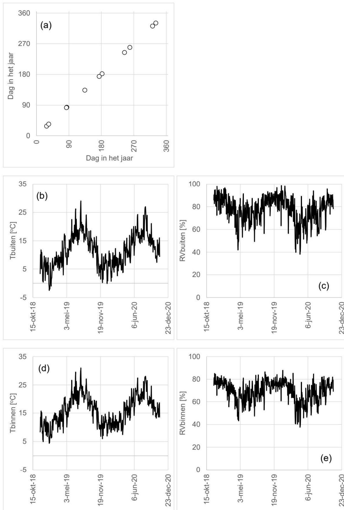
Figuur G1.1 a) Verdeling van de metingen over de seizoenen; b) t/m e) Continue metingen van een aantal klimaatparameters. T: temperatuur; RV: relatieve vochtigheid.
