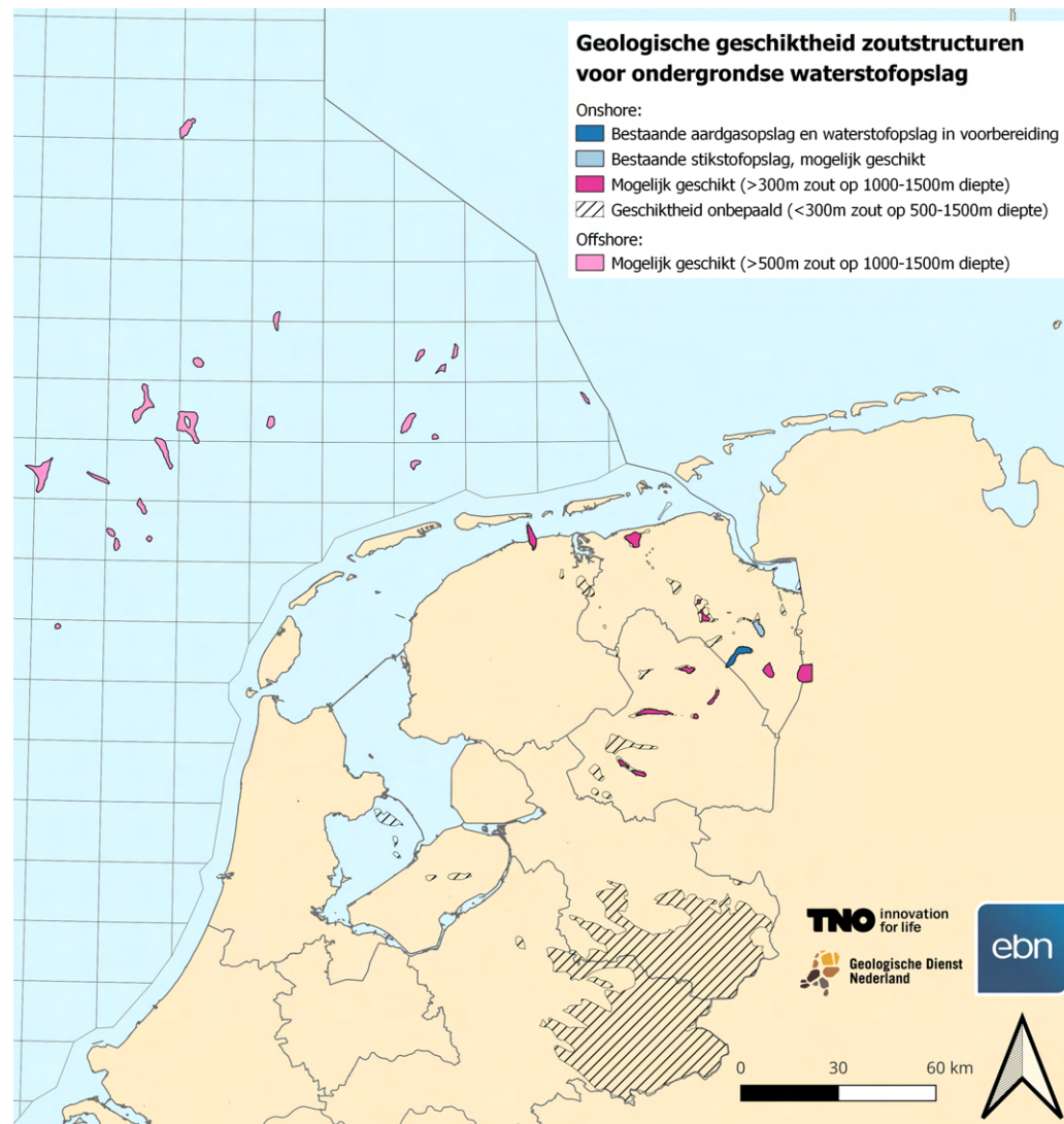
Figuur 6: Weergave van de zoutstructuren in Nederland die mogelijk geschikt (roze) zijn voor de ontwikkeling van cavernes voor ondergrondse waterstofopslag (UHS = Underground Hydrogen Storage) (bron: EBN & TNO).
