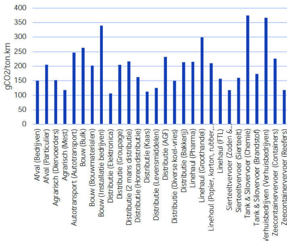
Figuur 5.2: CO 2 -uitstoot in gram per tonkilometer voor de segmenten volgens de Transport Performance Database.
