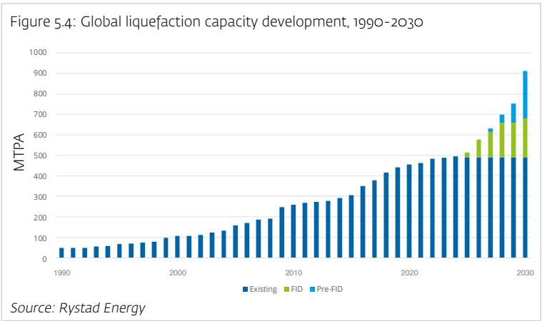
F IGUUR 8 Indicatie van de toename in de wereldwijde LNG-productiecapaciteit tot en met 2030 22 uitgesplitst naar “bestaand”, “FID” en “pre-FID”.
