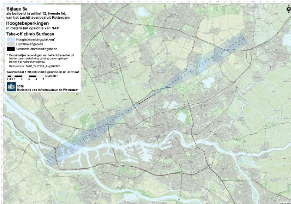
Bijlage 5a als bedoeld in artikel 12, tweede lid, van het Luchthavenbesluit Rotterdam Kaart (1:50.000) met hoogtebeperkingen: Take-off climb Surfaces
