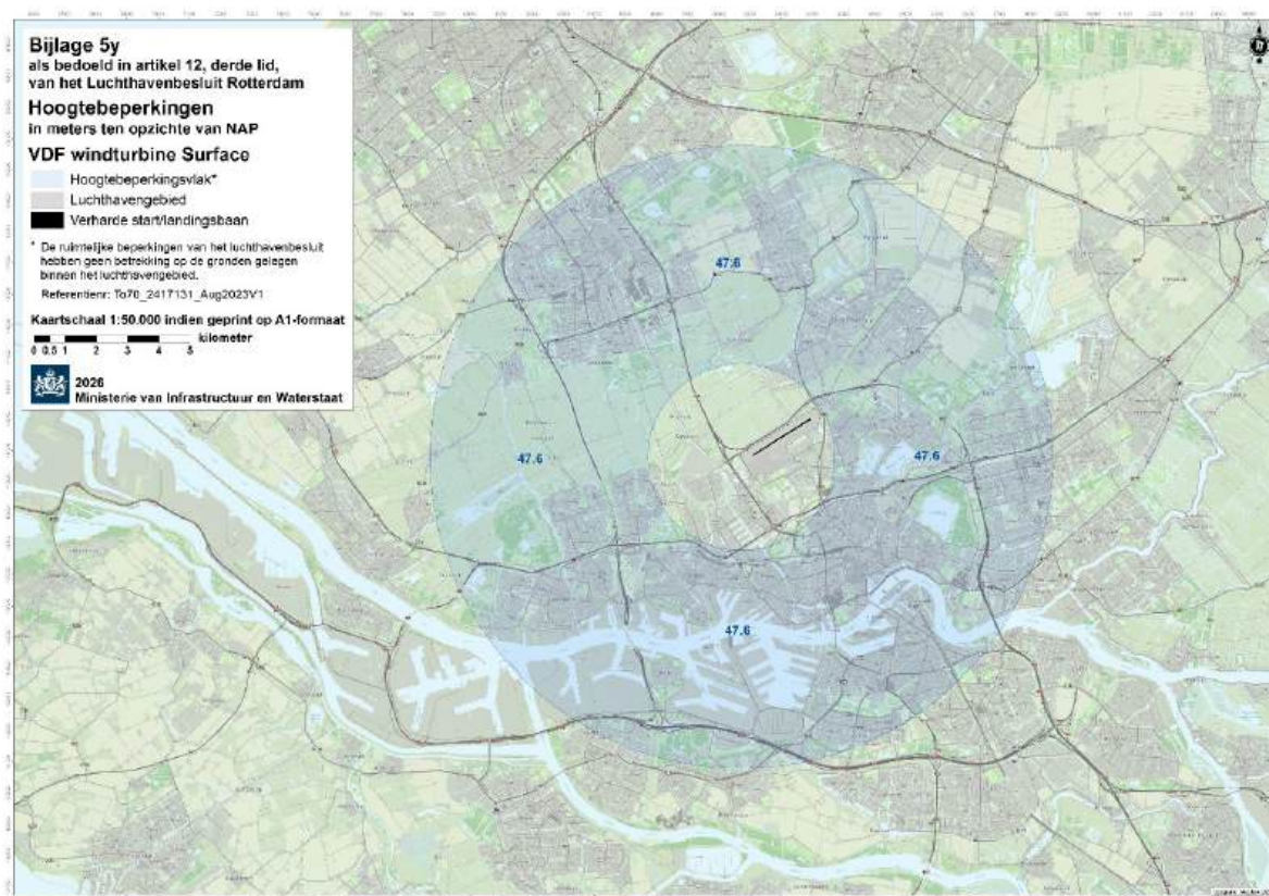
Bijlage 5y als bedoeld in artikel 12, derde lid, van het Luchthavenbesluit Rotterdam Kaart (1:50.000) met hoogtebeperkingen: Windturbine-surface voor de VDF-peiler
