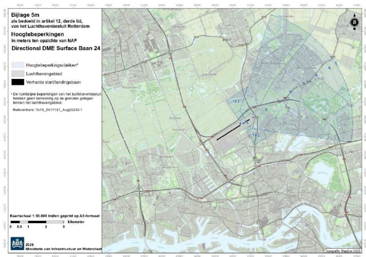
Bijlage 5m als bedoeld in artikel 12, derde lid, van het Luchthavenbesluit Rotterdam Kaart (1:50.000) met hoogtebeperkingen: Directional DME surface voor baan 24
