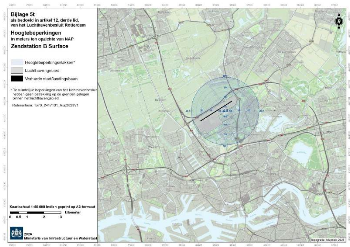
Bijlage 5t als bedoeld in artikel 12, derde lid, van het Luchthavenbesluit Rotterdam Kaart (1:50.000) met hoogtebeperkingen: Surface voor zendstation B
