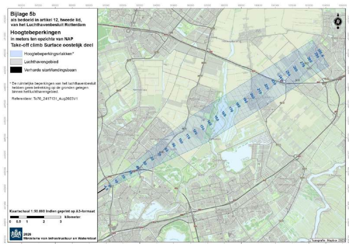
Bijlage 5b als bedoeld in artikel 12, tweede lid, van het Luchthavenbesluit Rotterdam Kaart (1:50.000) met hoogtebeperkingen: Take-off climb Surface oostelijk deel
