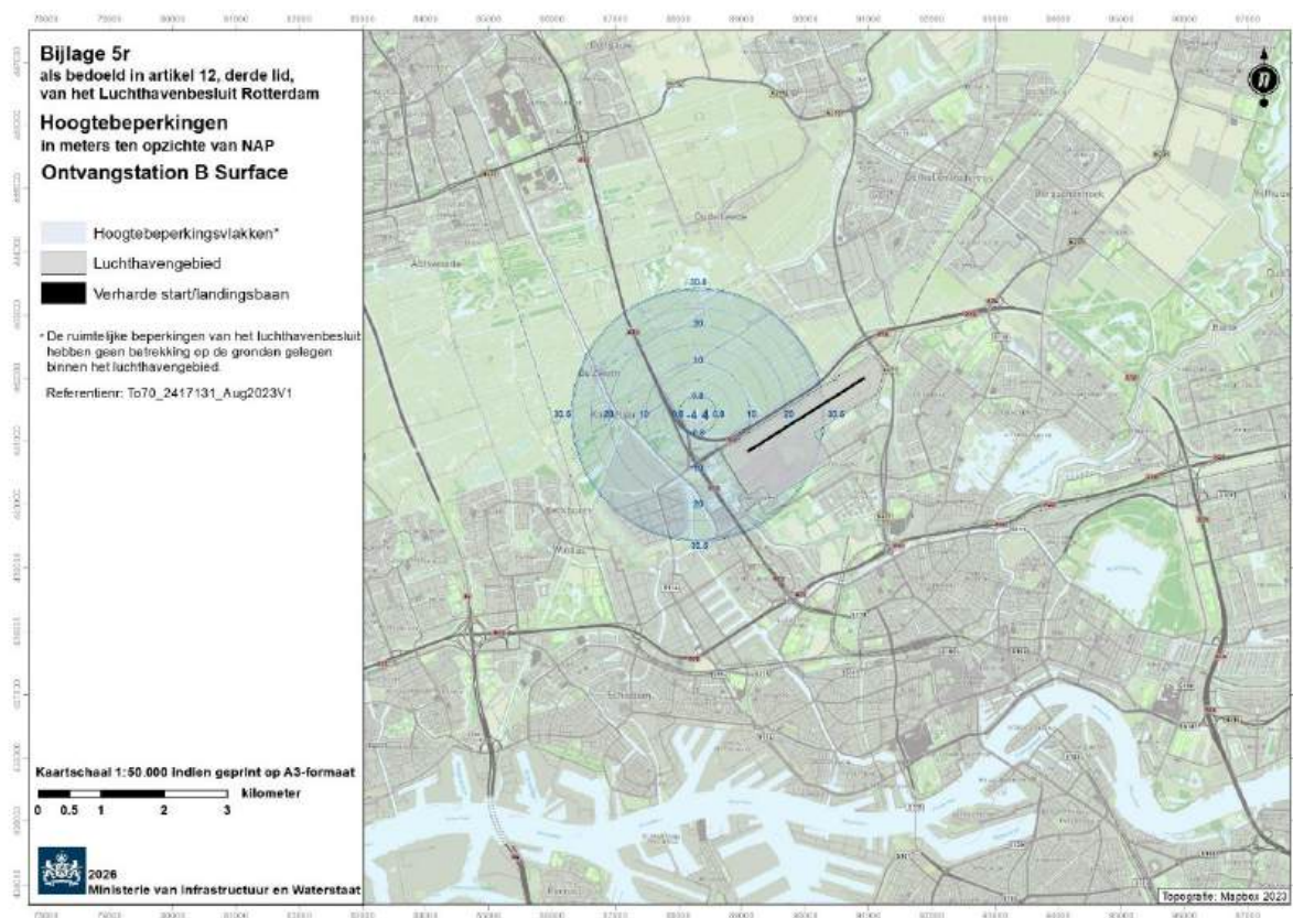
Bijlage 5r als bedoeld in artikel 12, derde lid, van het Luchthavenbesluit Rotterdam Kaart (1:50.000) met hoogtebeperkingen: Surface voor ontvangststation B
