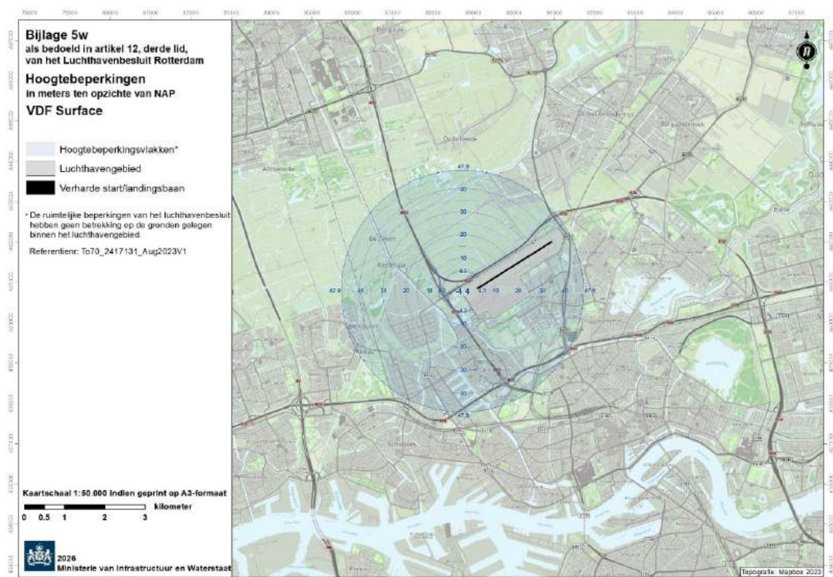
Bijlage 5w als bedoeld in artikel 12, derde lid, van het Luchthavenbesluit Rotterdam Kaart (1:50.000) met hoogtebeperkingen: Surface voor de VDF-peiler
