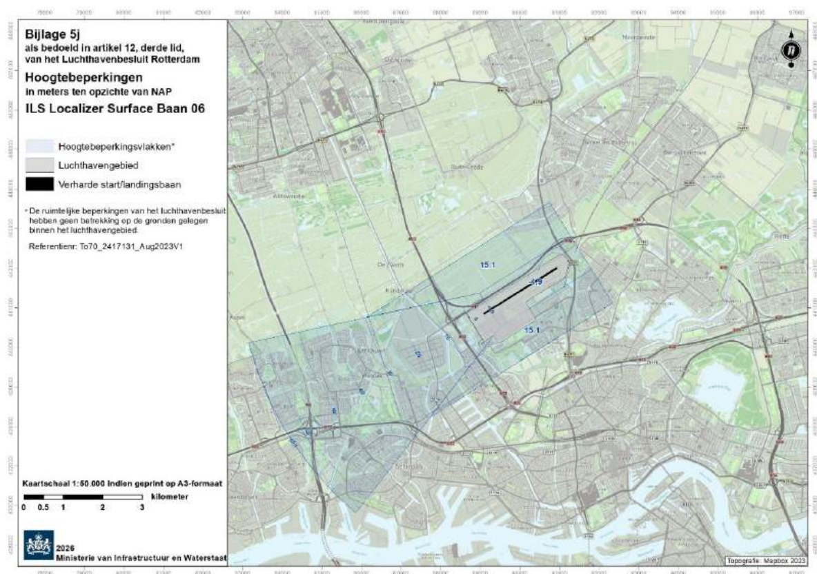
Bijlage 5j als bedoeld in artikel 12, derde lid, van het Luchthavenbesluit Rotterdam Kaart (1:50.000) met hoogtebeperkingen: ILS-surface voor baan 06
