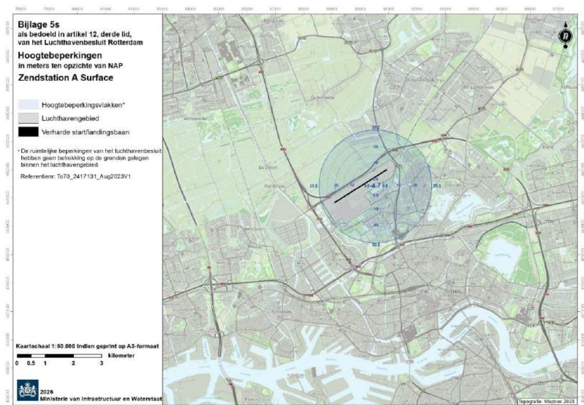
Bijlage 5s als bedoeld in artikel 12, derde lid, van het Luchthavenbesluit Rotterdam Kaart (1:50.000) met hoogtebeperkingen: Surface voor zendstation A
