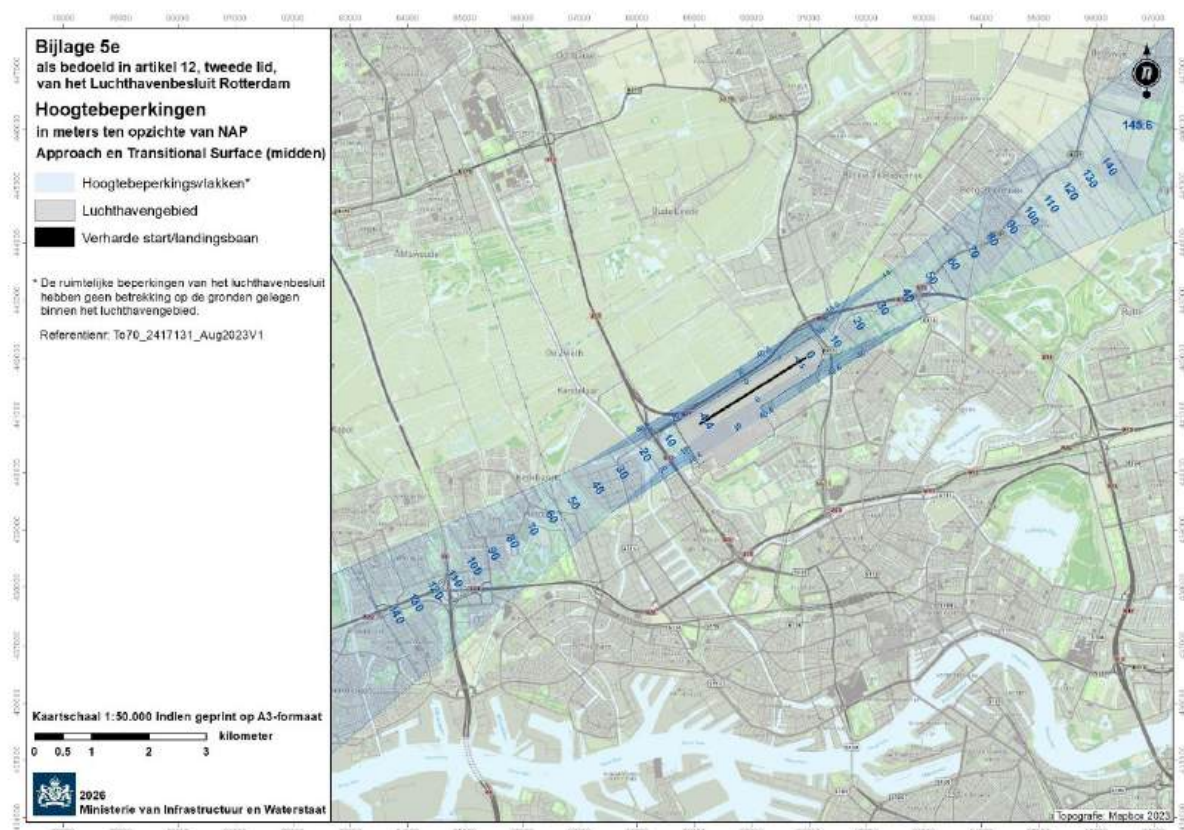
Bijlage 5e als bedoeld in artikel 12, tweede lid, van het Luchthavenbesluit Rotterdam Kaart (1:50.000) met hoogtebeperkingen: Approach en Transitional Surfaces middendeel
