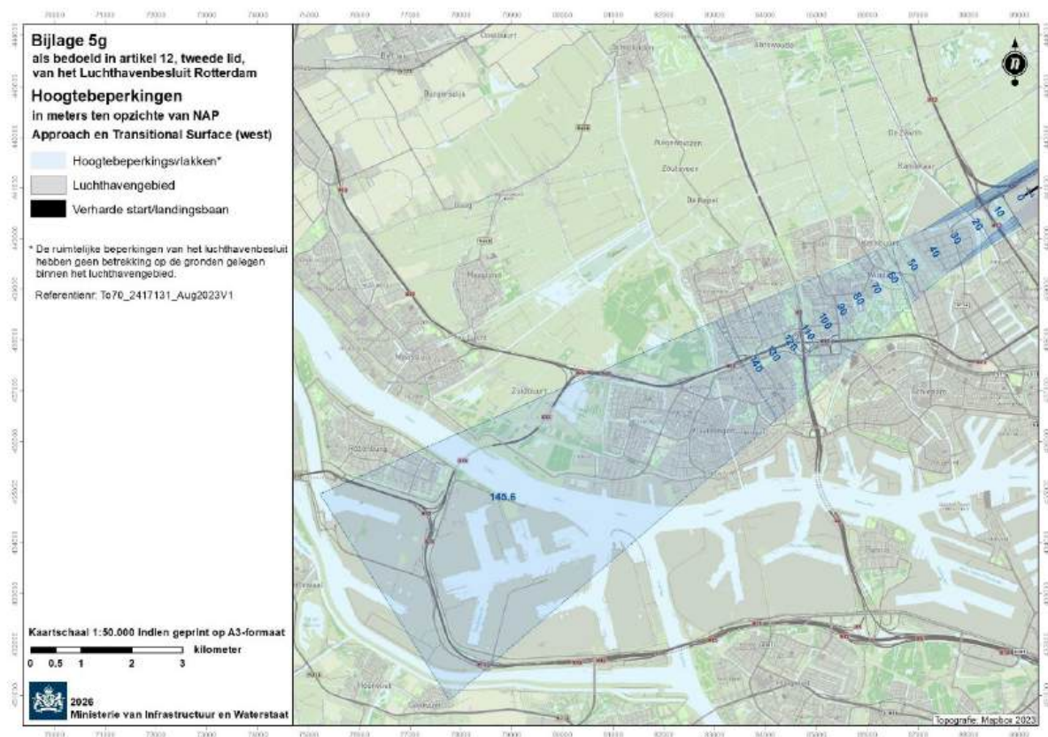
Bijlage 5g als bedoeld in artikel 12, tweede lid, van het Luchthavenbesluit Rotterdam Kaart (1:50.000) met hoogtebeperkingen: Approach en Transitional Surfaces westelijk deel
