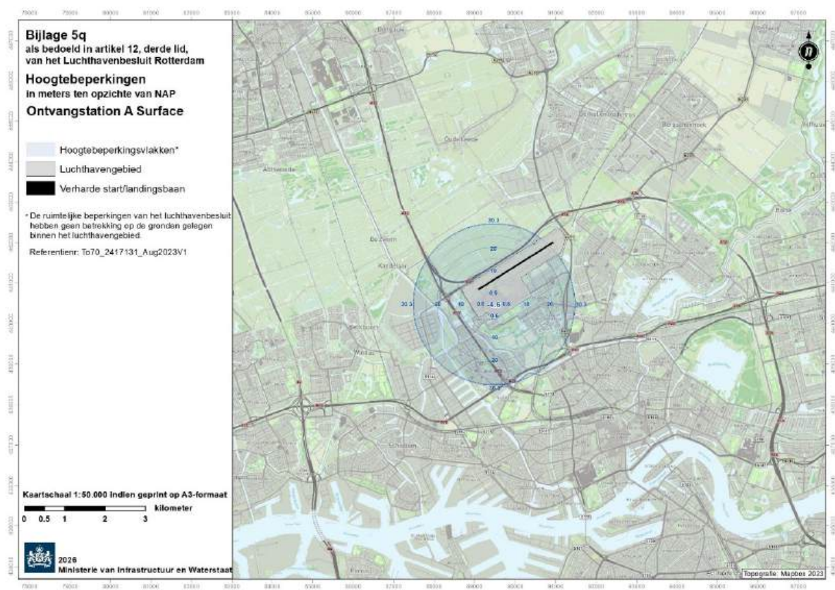
Bijlage 5q als bedoeld in artikel 12, derde lid, van het Luchthavenbesluit Rotterdam Kaart (1:50.000) met hoogtebeperkingen: Surface voor ontvangststation A
