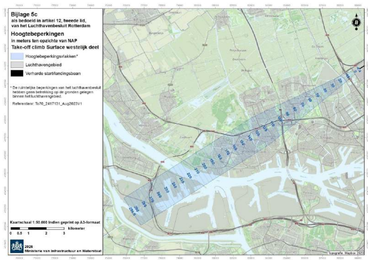
Bijlage 5c als bedoeld in artikel 12, tweede lid, van het Luchthavenbesluit Rotterdam Kaart (1:50.000) met hoogtebeperkingen: Take-off climb Surface westelijk deel
