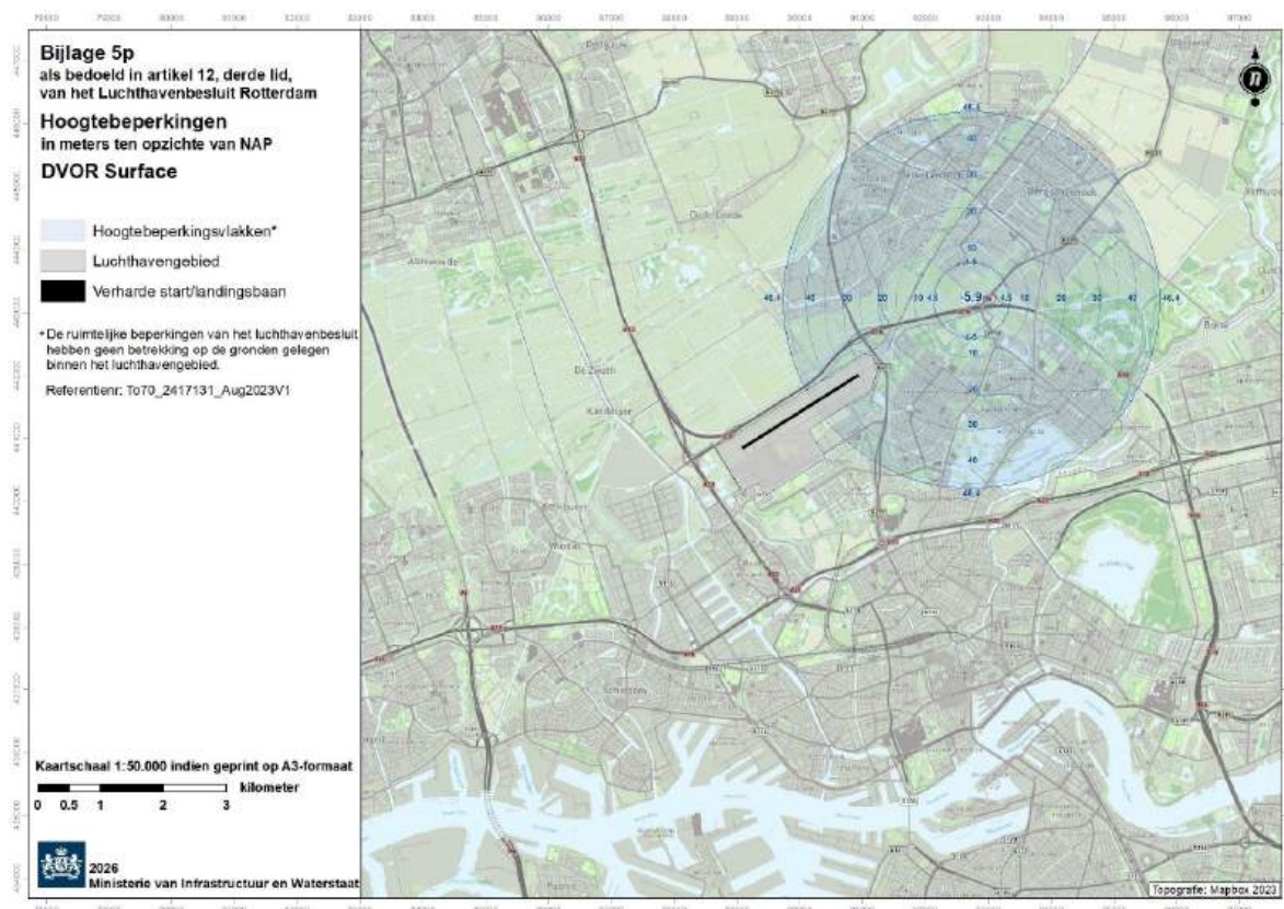
Bijlage 5p als bedoeld in artikel 12, derde lid, van het Luchthavenbesluit Rotterdam Kaart (1:50.000) met hoogtebeperkingen: Surface voor de DVOR
