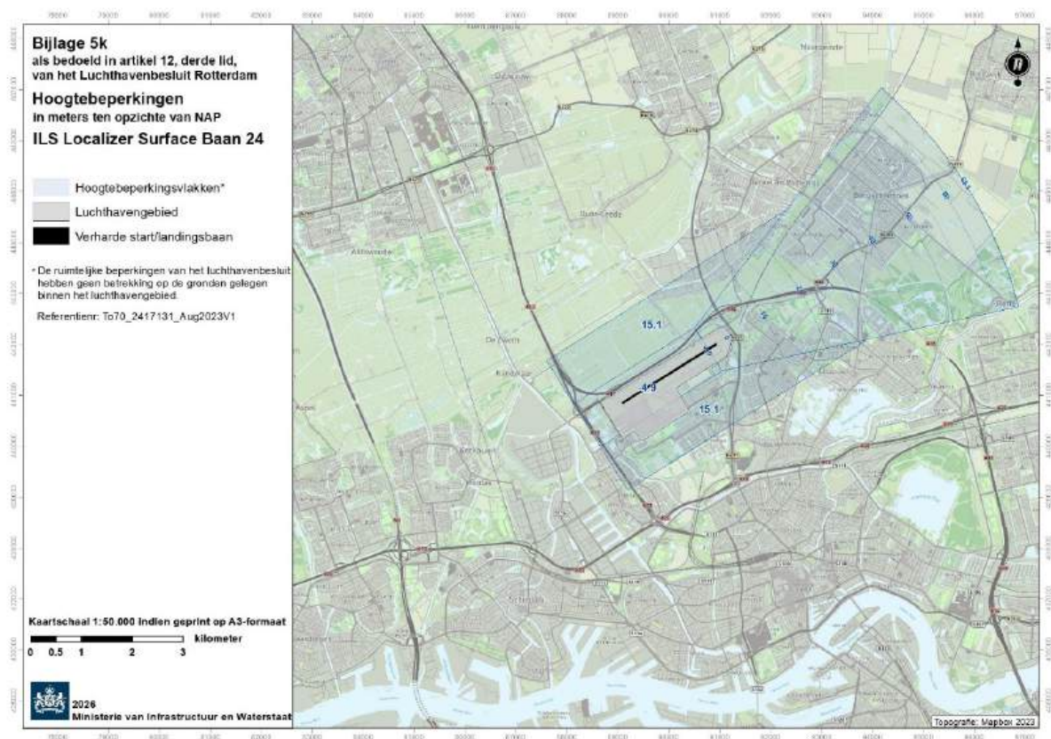
Bijlage 5k als bedoeld in artikel 12, derde lid, van het Luchthavenbesluit Rotterdam Kaart (1:50.000) met hoogtebeperkingen: ILS-surface voor baan 24
