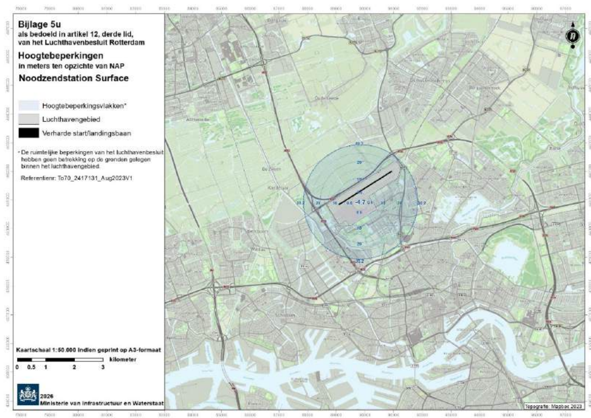
Bijlage Su als bedoeld in artikel 12, derde lid, van het Luchthavenbesluit Rotterdam Kaart (1:50.000) met hoogtebeperkingen: Surface voor noodzendstation
