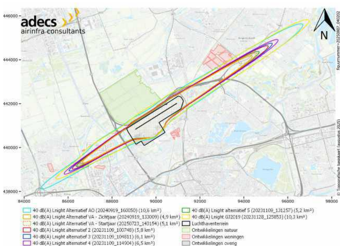
Figuur 33 Vergelijking van 40 dB(A) L_{\text{night}} -contouren van alle alternatieven.
